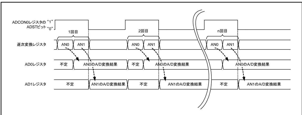
図 3.2 単掃引モード動作図
