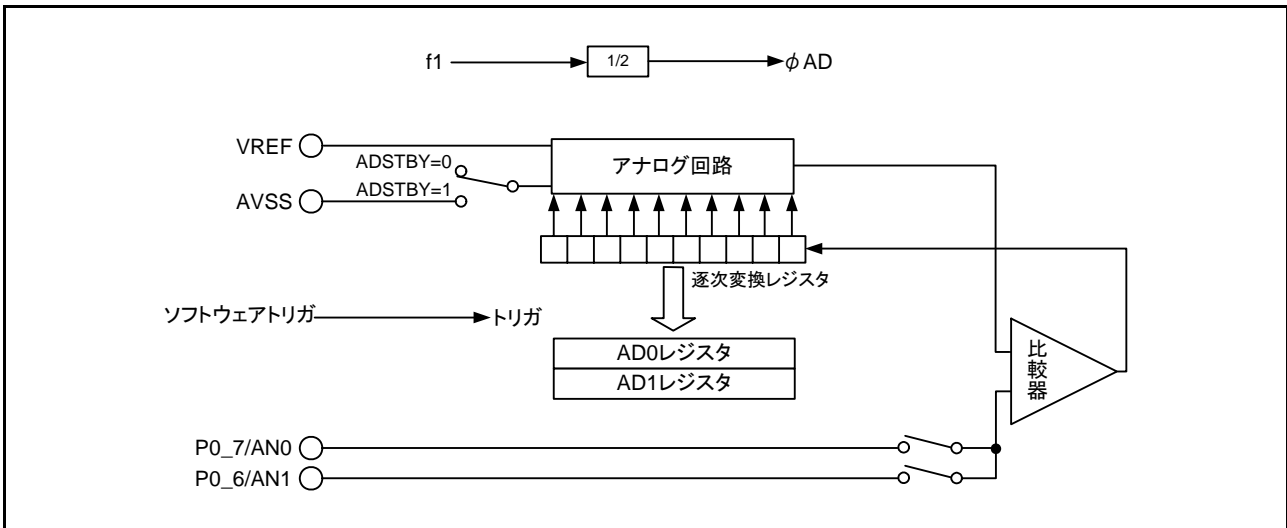
図 3.1 ブロック図
