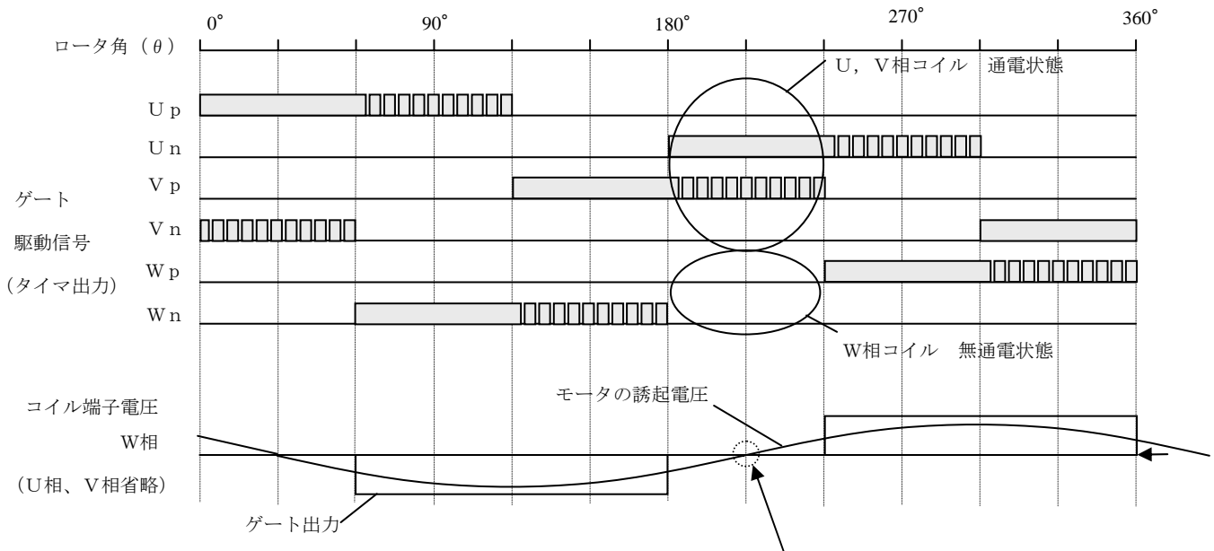
▼ 図3. 4. 6 位置センサレス120度矩形波制御
