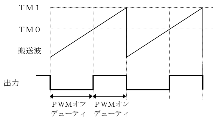
▼ 図3.3.5 PWMデューティ
