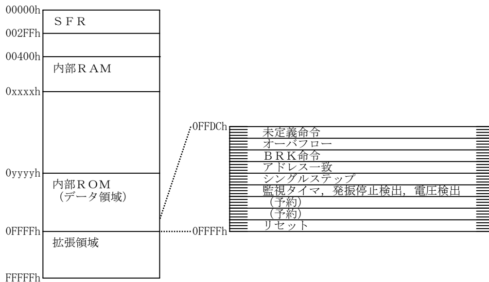
▼ 図 3. 3. 7 メモリ配置
