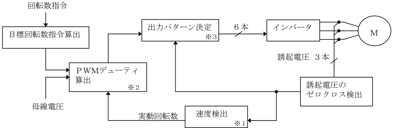
▼ 図3. 3. 2 制御ブロック図
