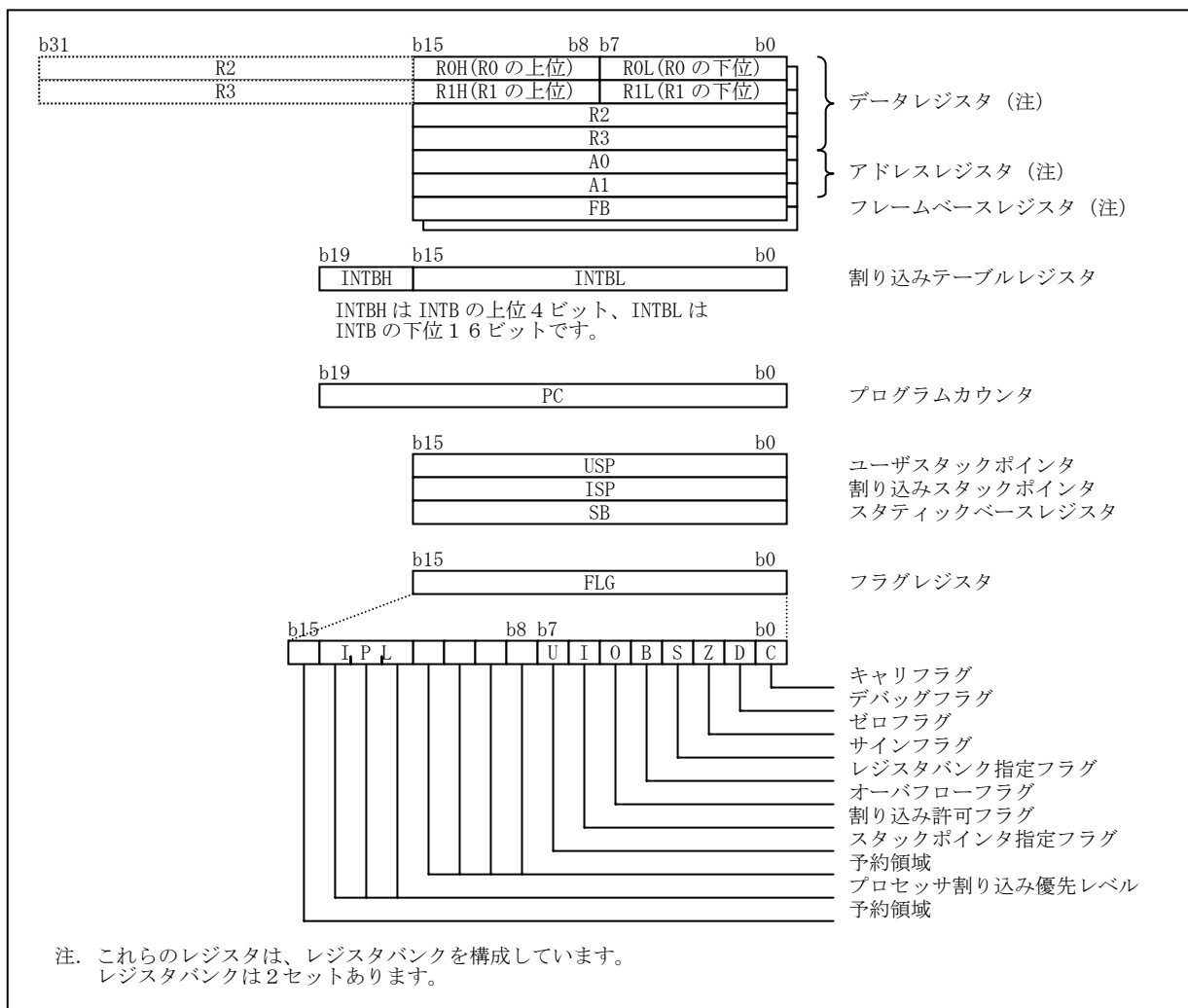
▼ 図 3. 3. 6 CPUのレジスタ
