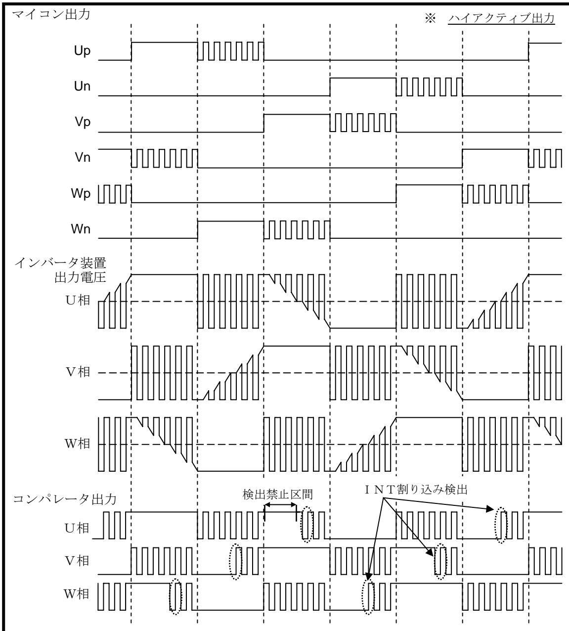
▼ 図 3. 3. 4 誘起電圧の検出方法
