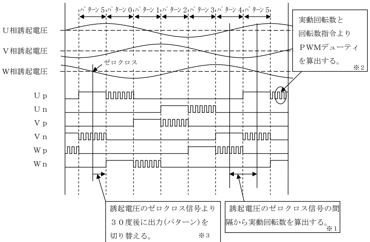
▼ 図3. 3. 3 タイミングチャート
