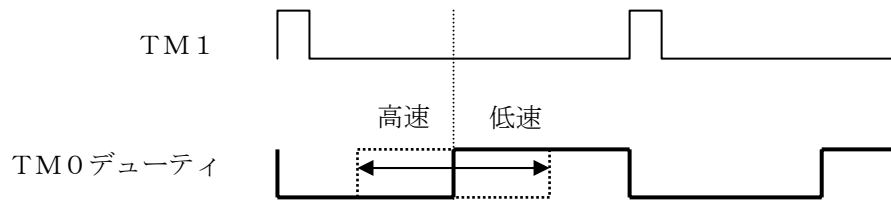
▼ 図3. 2. 6 回転数指令値とTM0の関係
