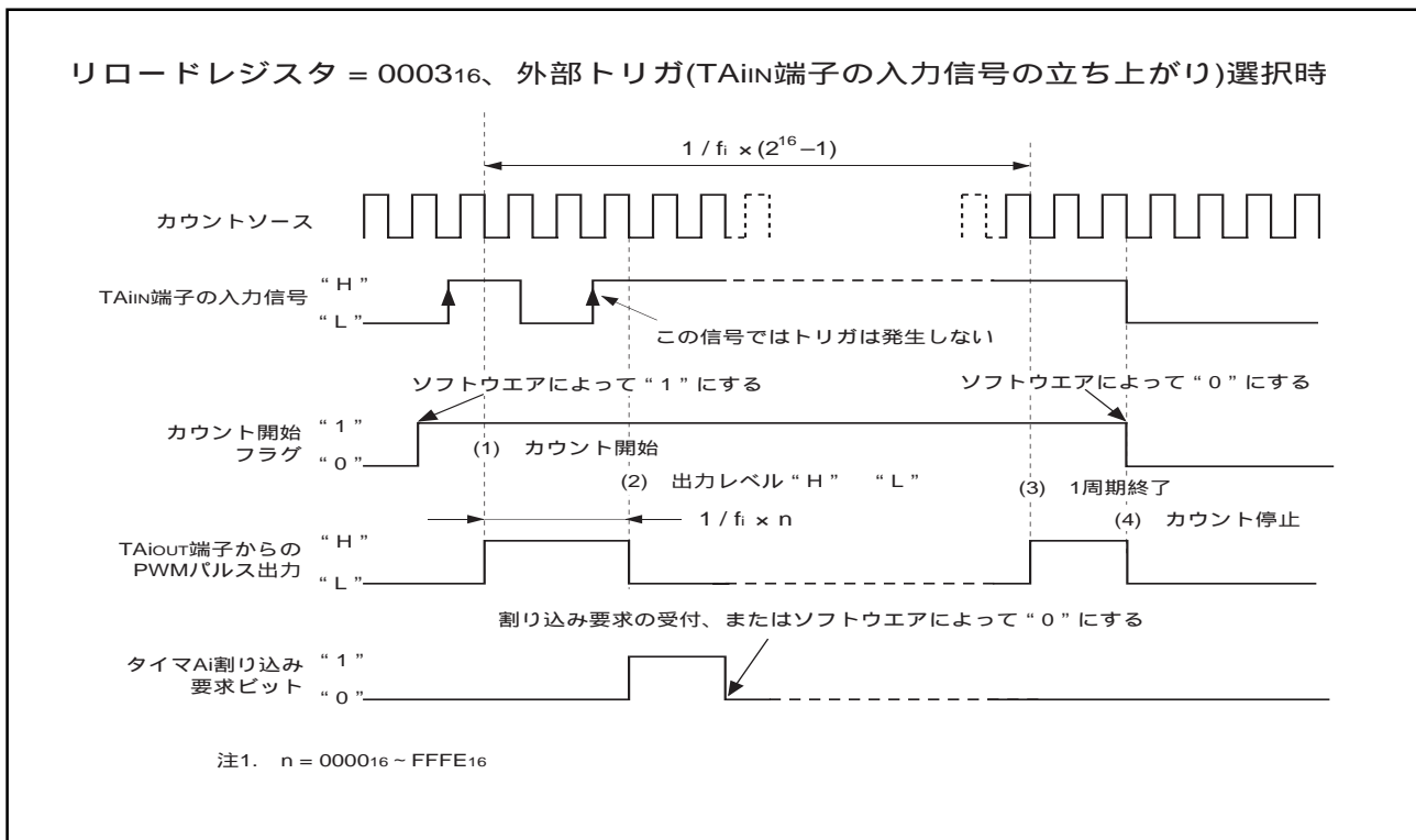
図1 パルス幅変調モード動作、16ビットPWMモード選択時のタイミング
