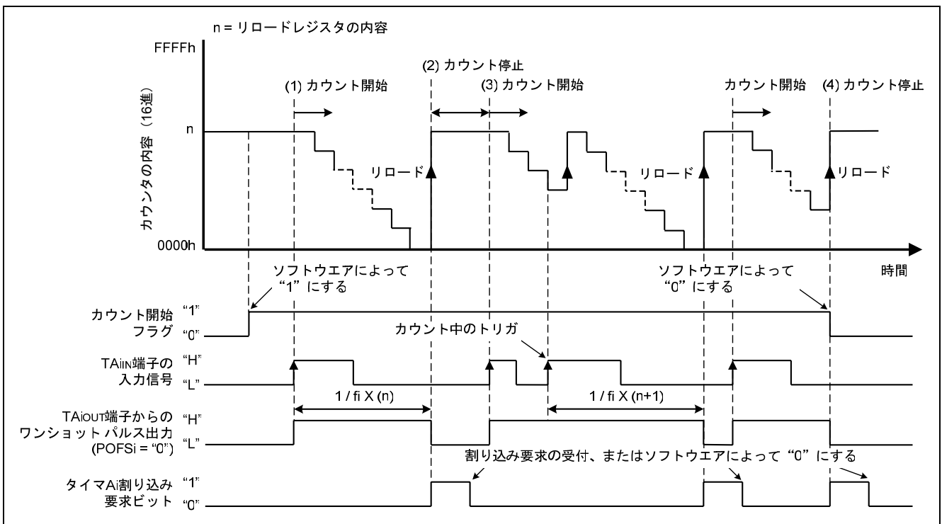
図1 ワンショットタイマモード、外部トリガ選択時の動作タイミング
