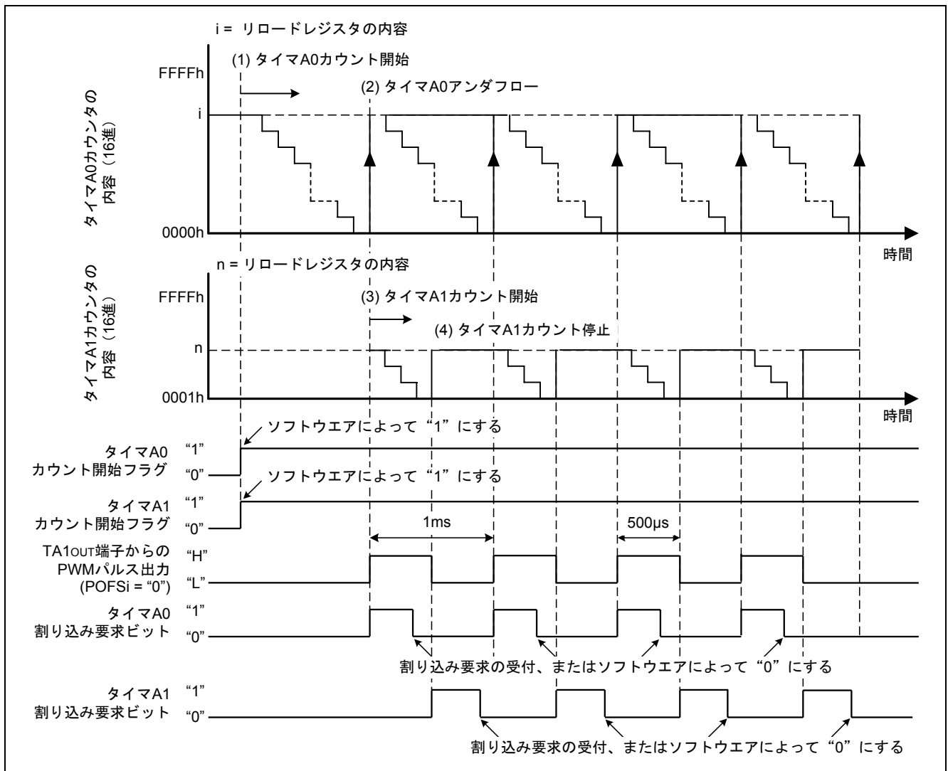
図 1. 周期およびデューティー可変の PWM 出力の動作タイミング
