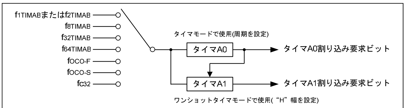
図 2. 周期およびデューティー可変の PWM 出力のタイマ接続図
