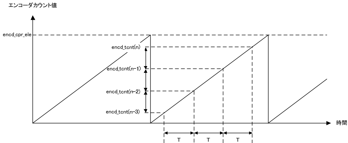
図 3-6 エンコーダ利用による速度演算
