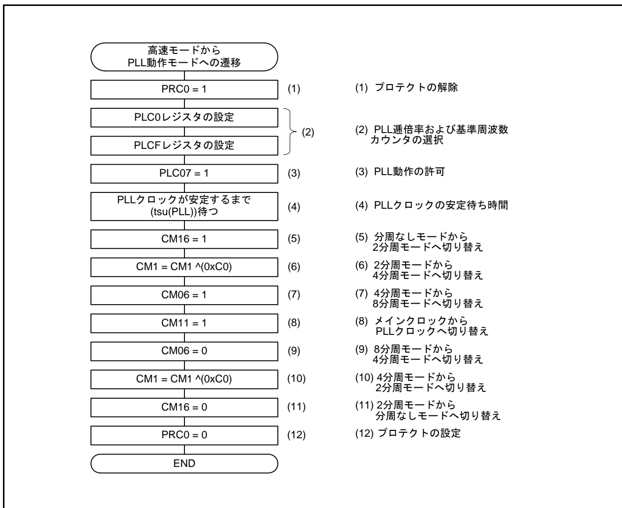
図3.1 高速モードからPLL動作モードへの遷移
