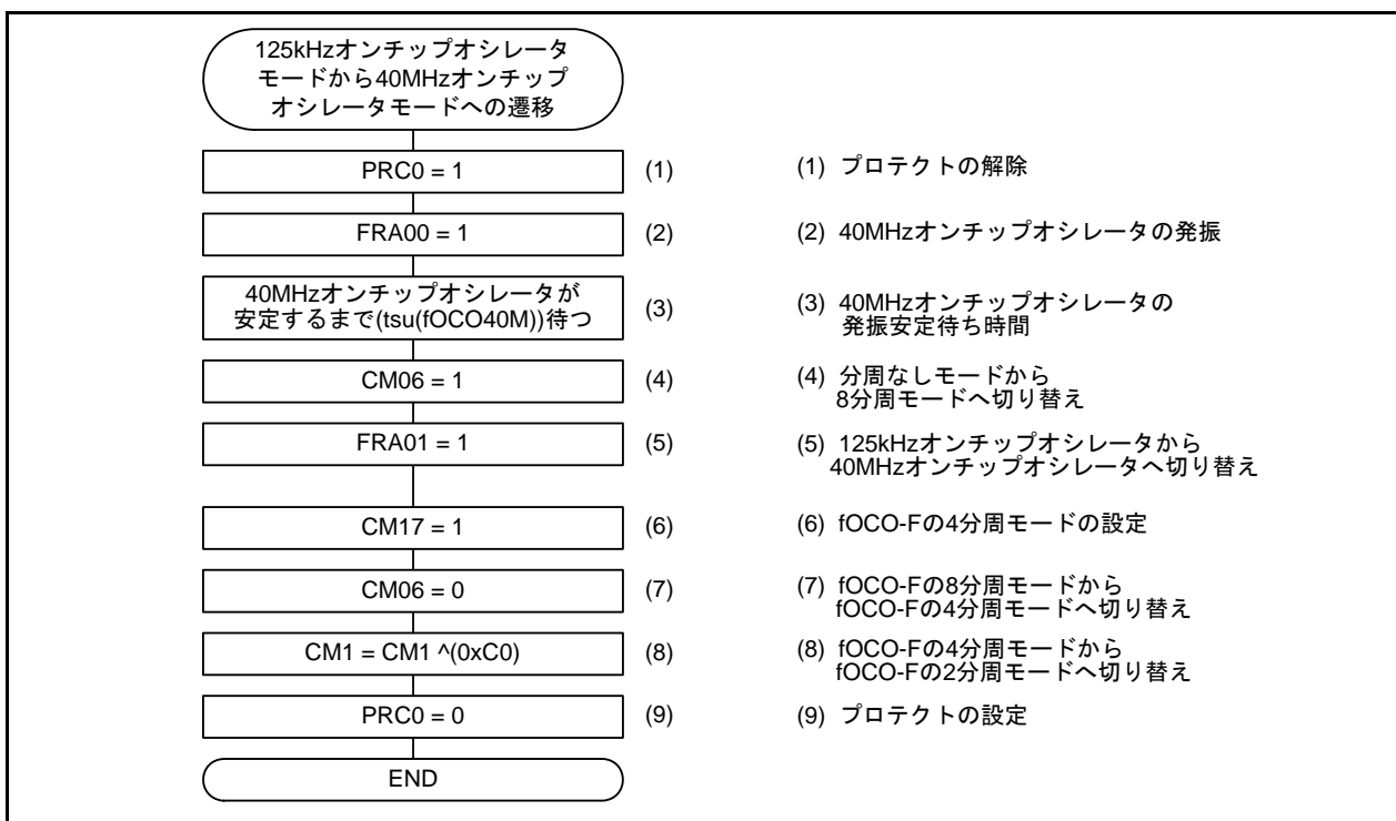
図3.5 125kHzオンチップオシレータモードから40MHzオンチップオシレータモード(fOCO-Fの2分周)への遷移
