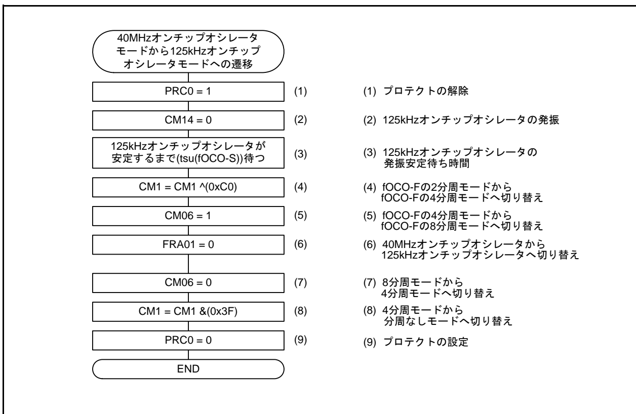
図3.2 40MHzオンチップオシレータモード(fOCO-Fの2分周)から125kHzオンチップオシレータモードへの遷移
