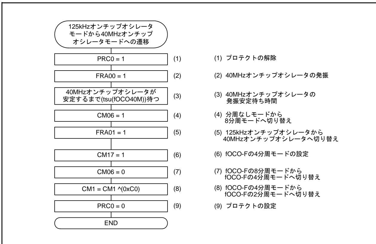
図3.7 125kHzオンチップオシレータモードから40MHzオンチップオシレータモードへの遷移
