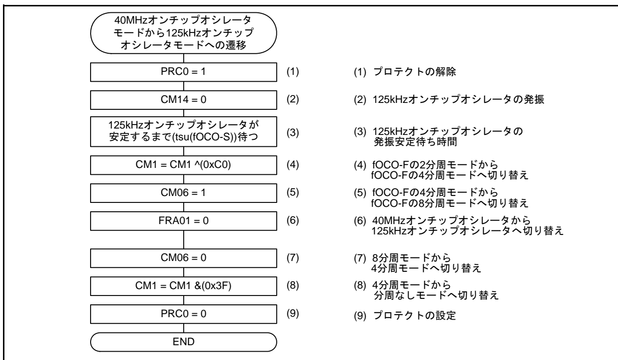
図3.2 40MHzオンチップオシレータモード(fOCO-Fの2分周)から125kHzオンチップオシレータモードへの遷移
