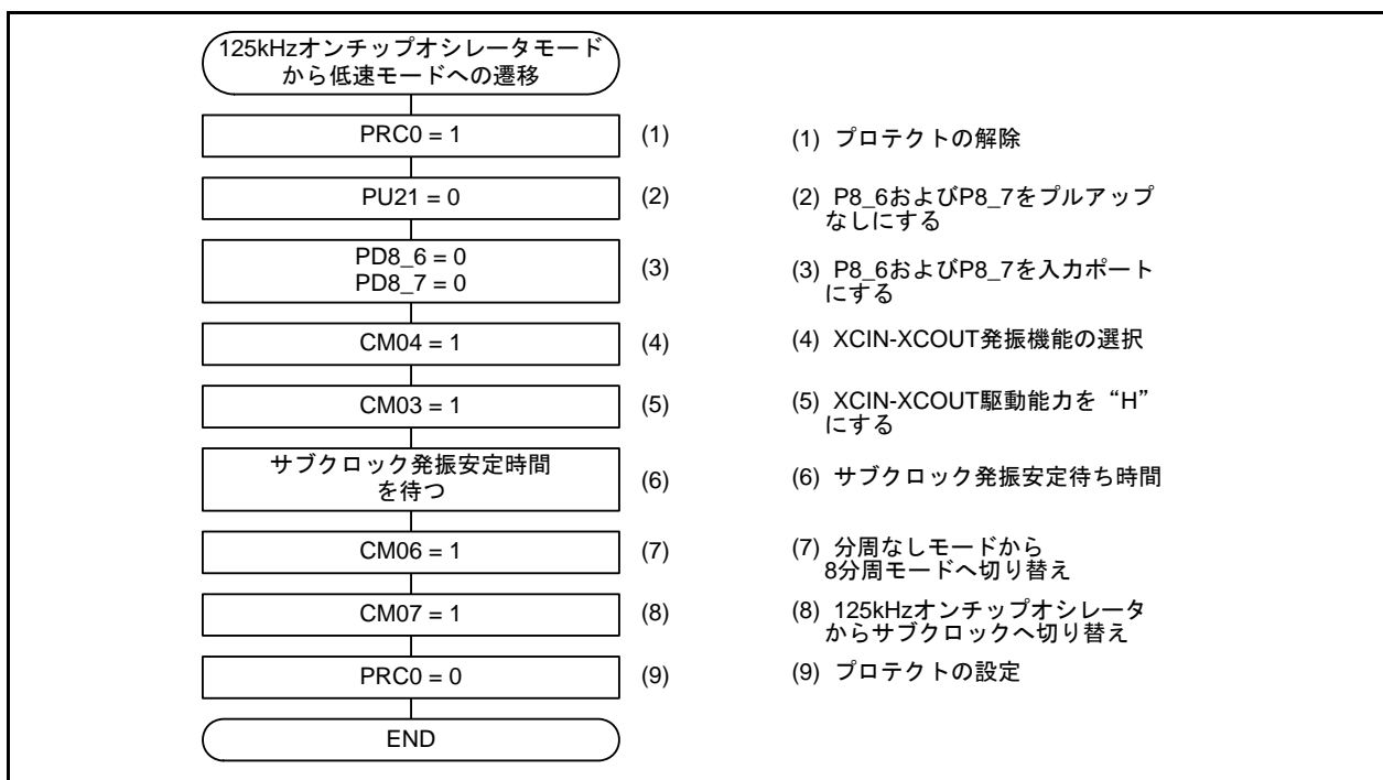
図3.3 125kHzオンチップオシレータモードから低速モードへの遷移
