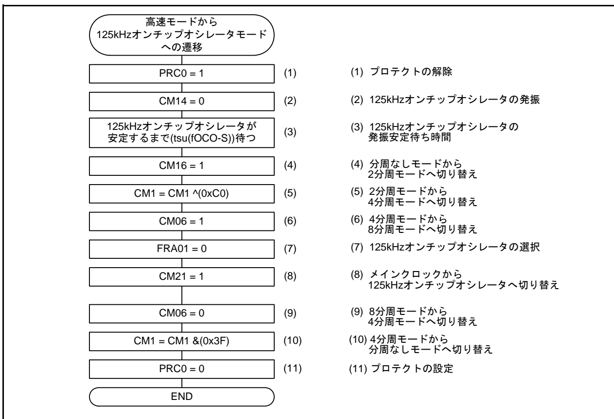
図3.2 高速モードから125kHzオンチップオシレータモードへの遷移
