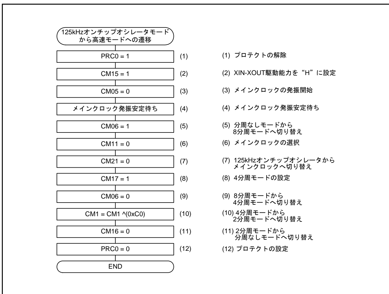
図3.5 125kHzオンチップオシレータモードから高速モードへの遷移
