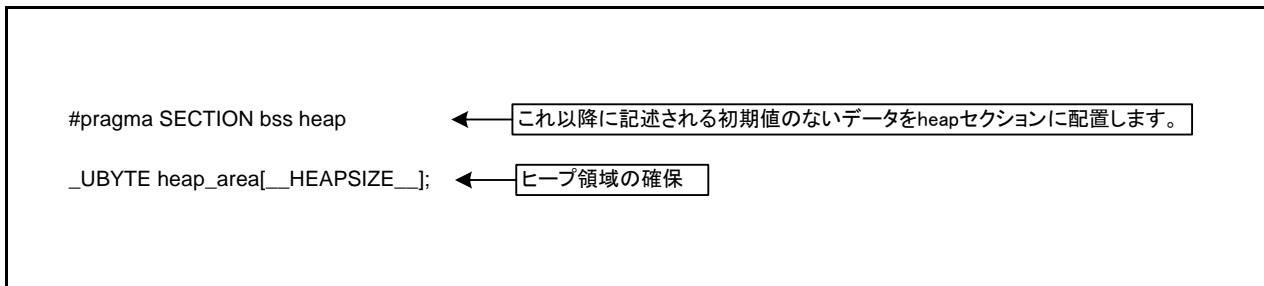
図 4.5 ヒープ領域の設定
