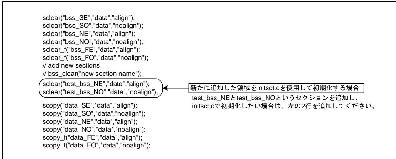
図 4.4 新たに追加した領域をinitsct.cを使用して初期化する例
