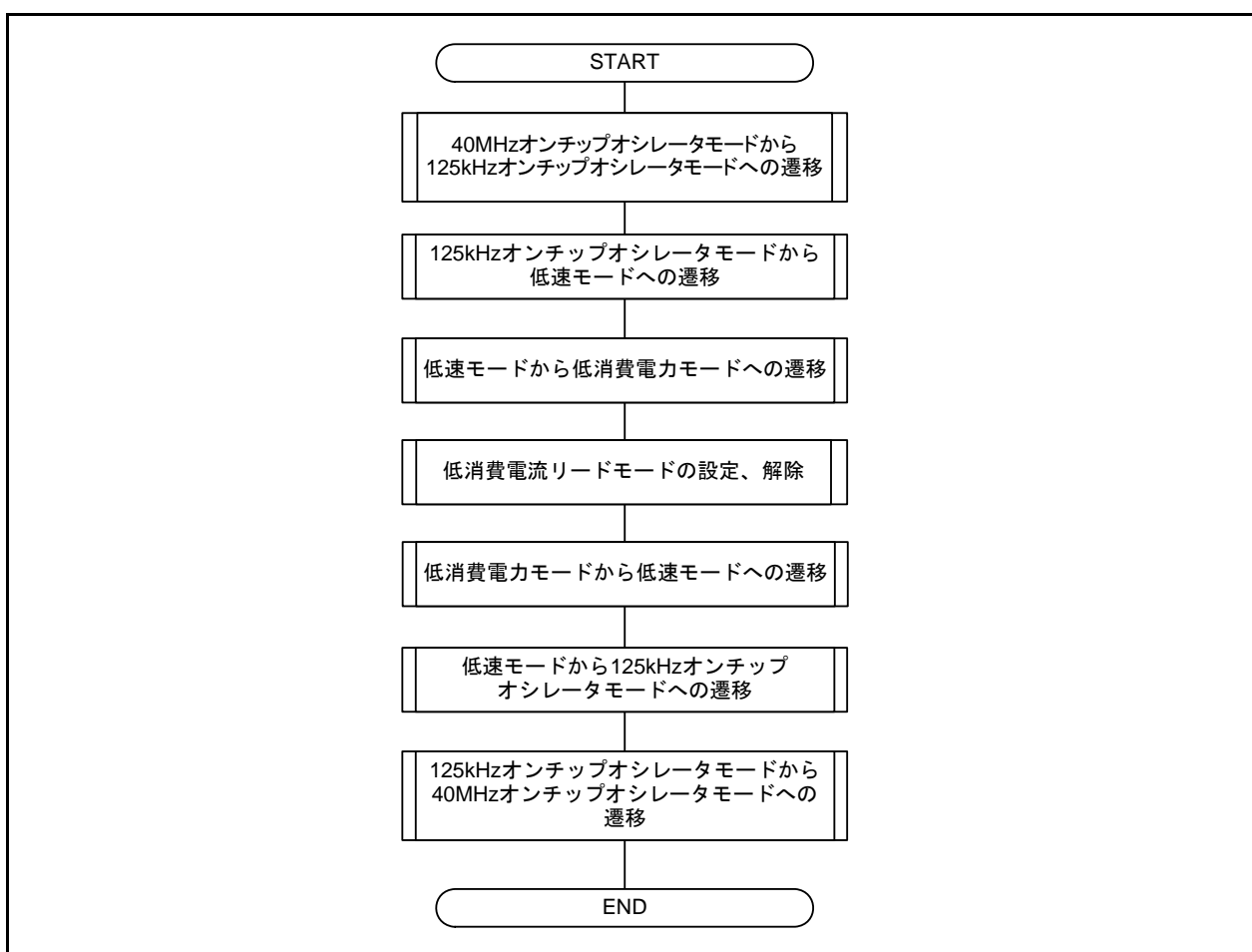
図3.1 40MHzオンチップオシレータモードと低消費電力モード間の遷移手順
