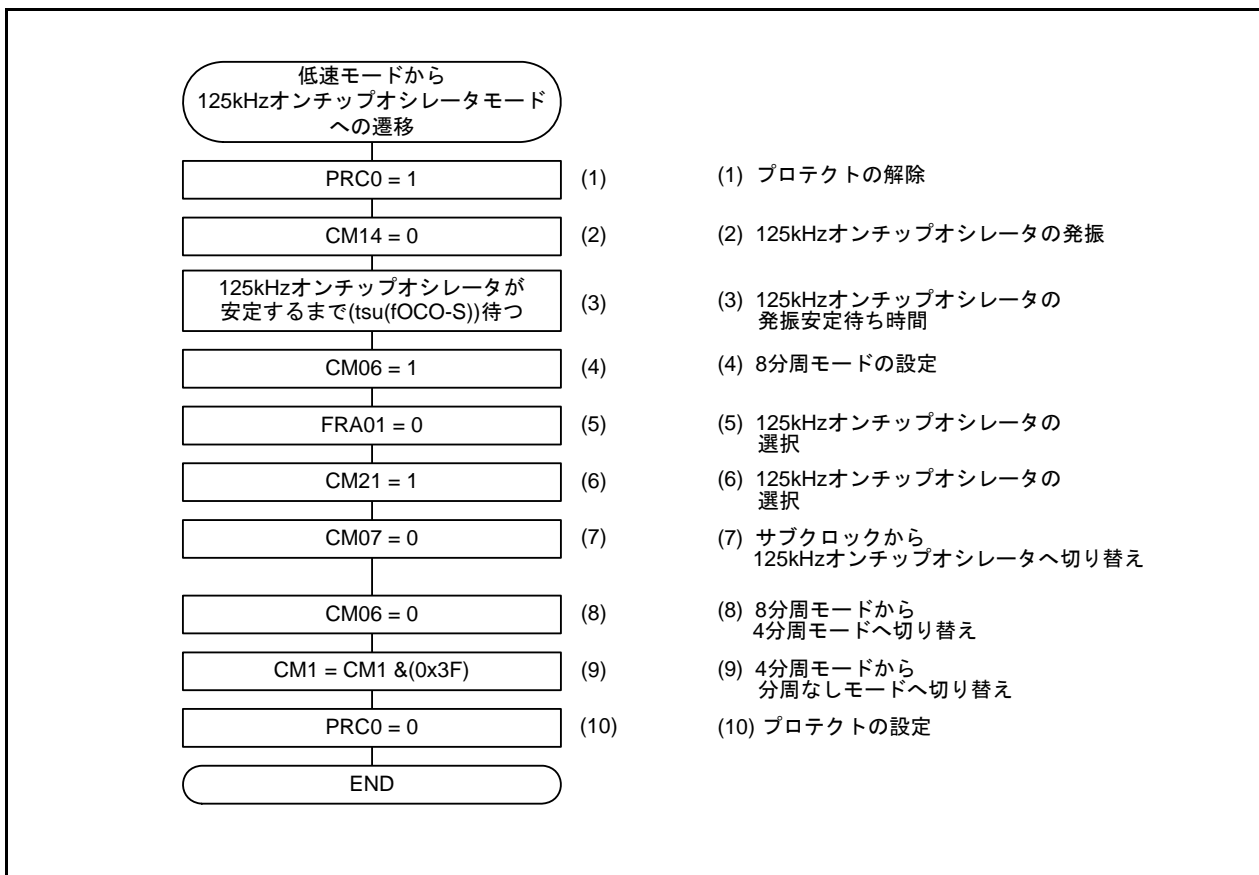
図3.6 低速度モードから125kHzオンチップオシレータモードへの遷移
