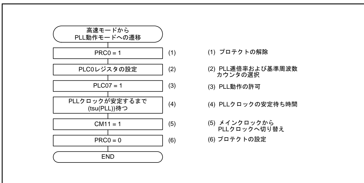
図3.1 高速モードからPLL動作モードへの遷移
