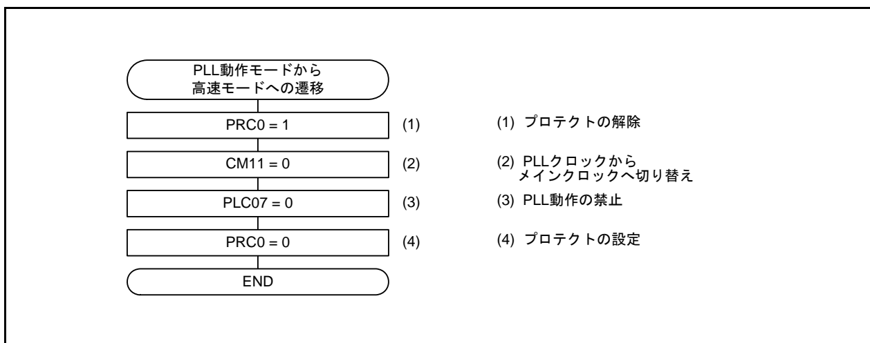
図3.2 PLL動作モードから高速モードへの遷移
