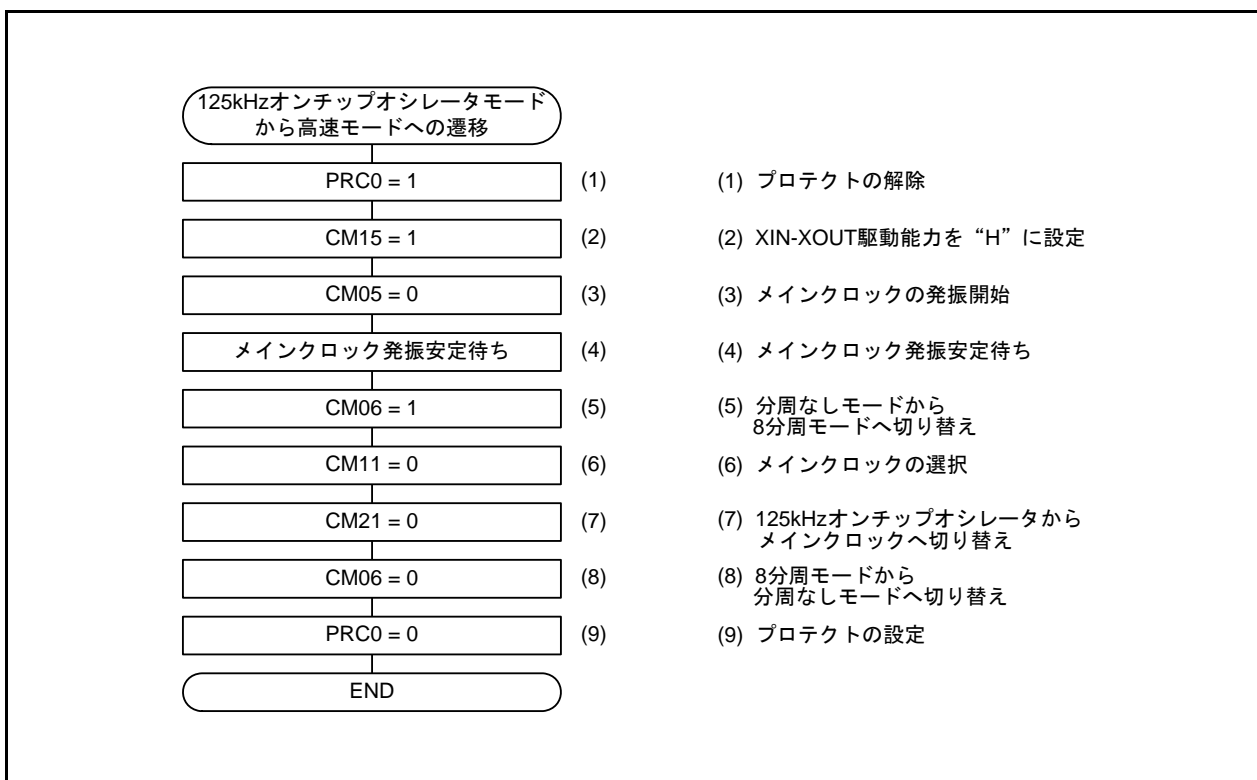
図 3.5 125kHz オンチップオシレータモードから高速モードへの遷移
