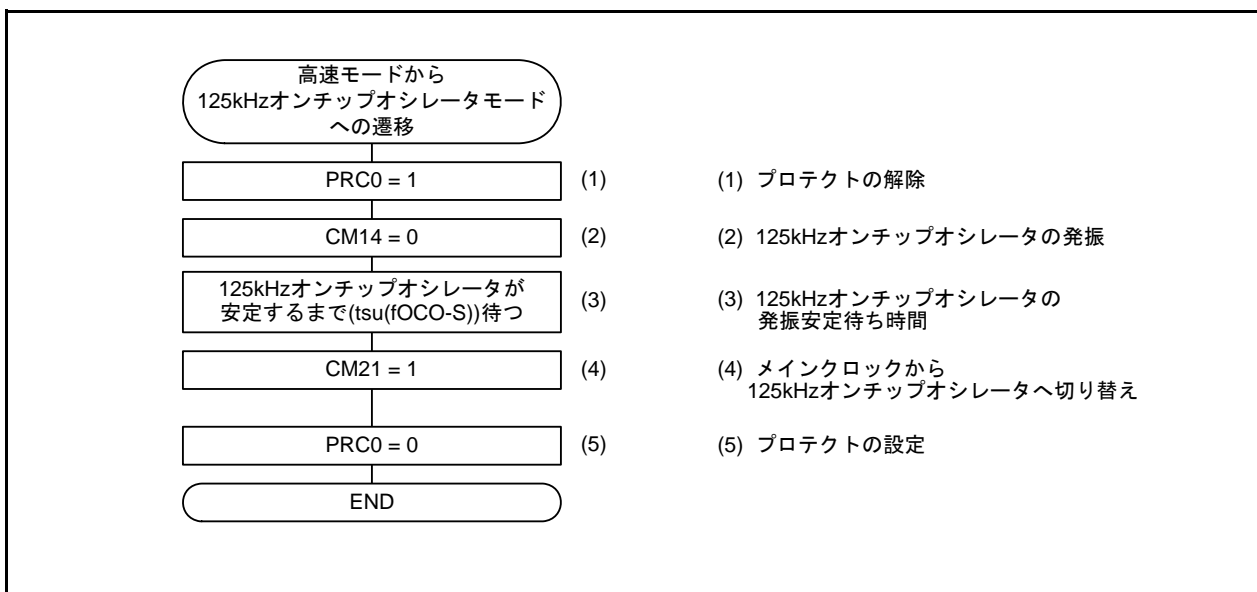
図3.2 高速モードから125kHzオンチップオシレータモードへの遷移
