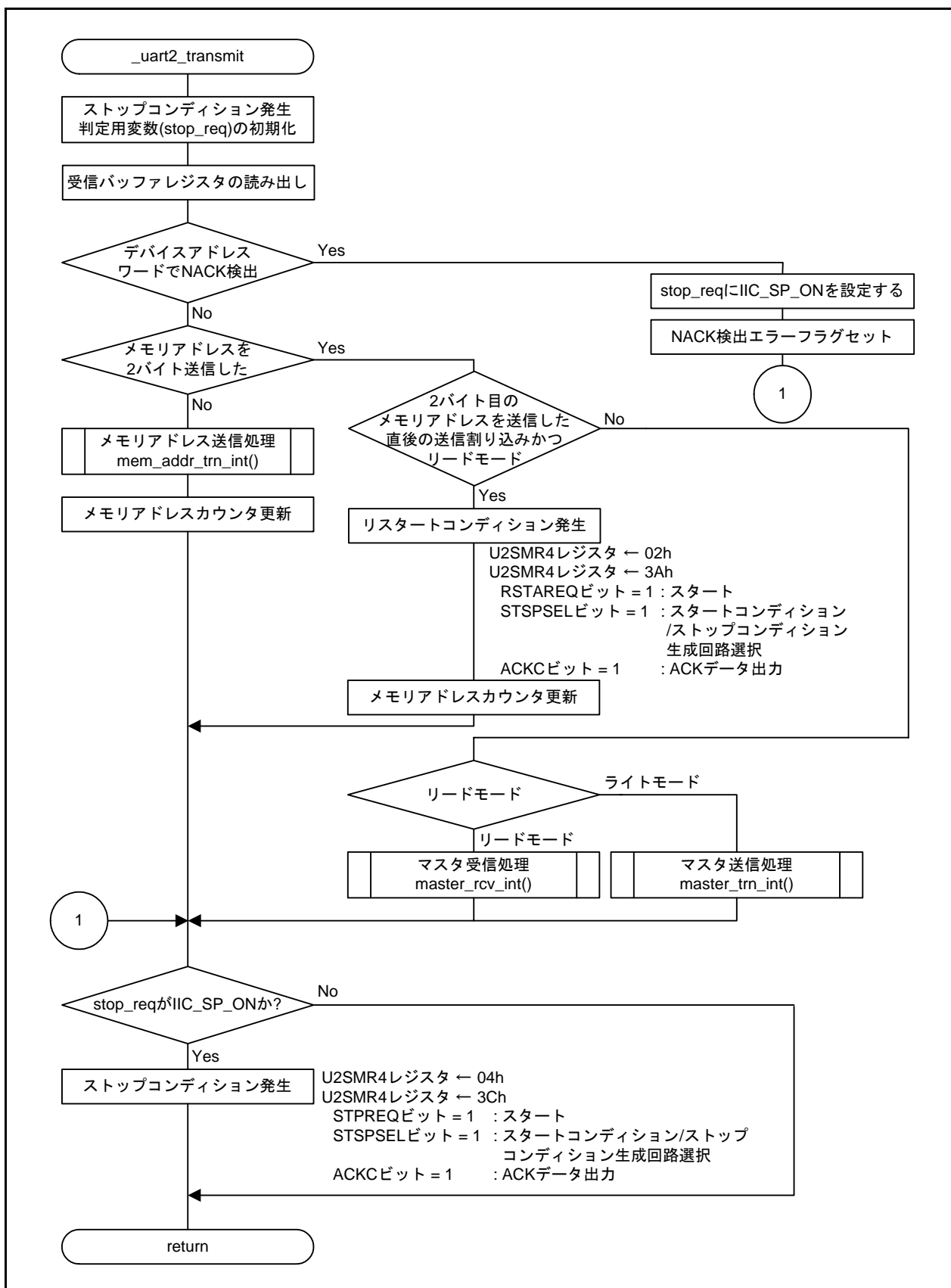
図 5.13 UART2送信割り込み処理
