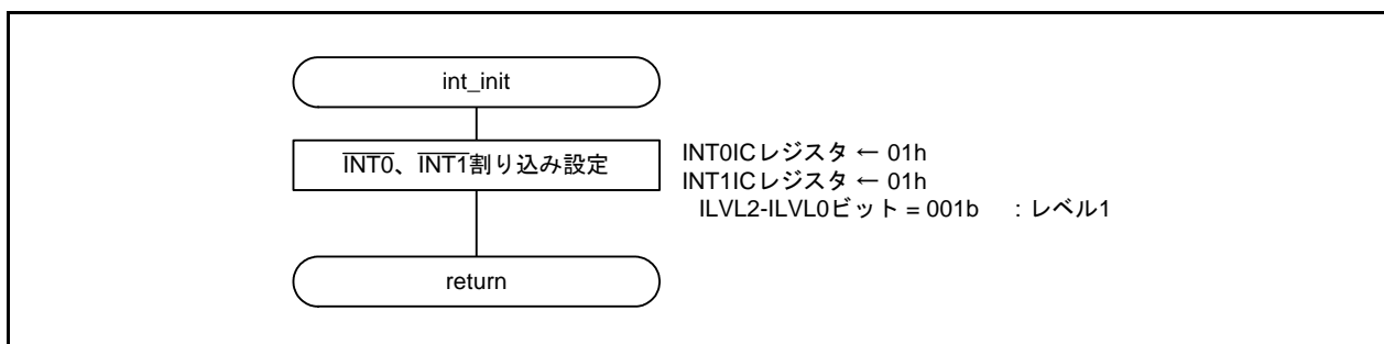
図 5.17 \overline{\text{INT0}} 、 \overline{\text{INT1}} 初期設定処理
