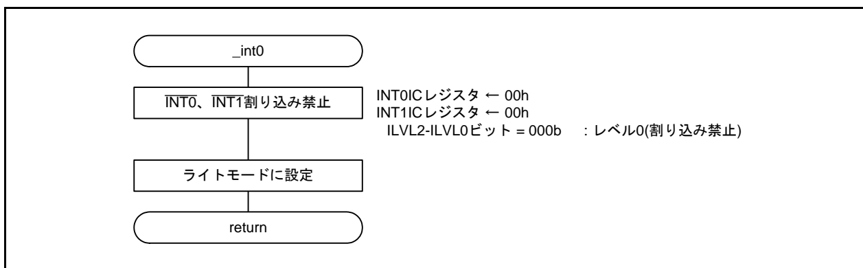
図 5.18 \overline{\text{INT0}} 割り込み処理
