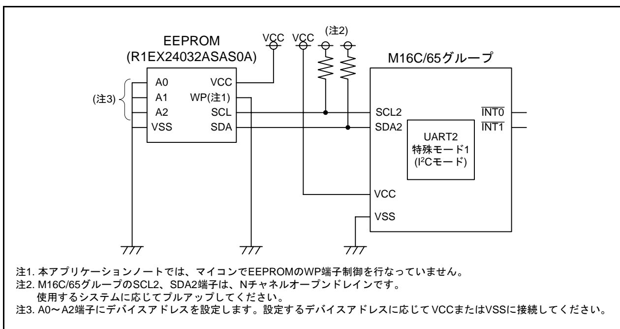
図 1.1 接続図
