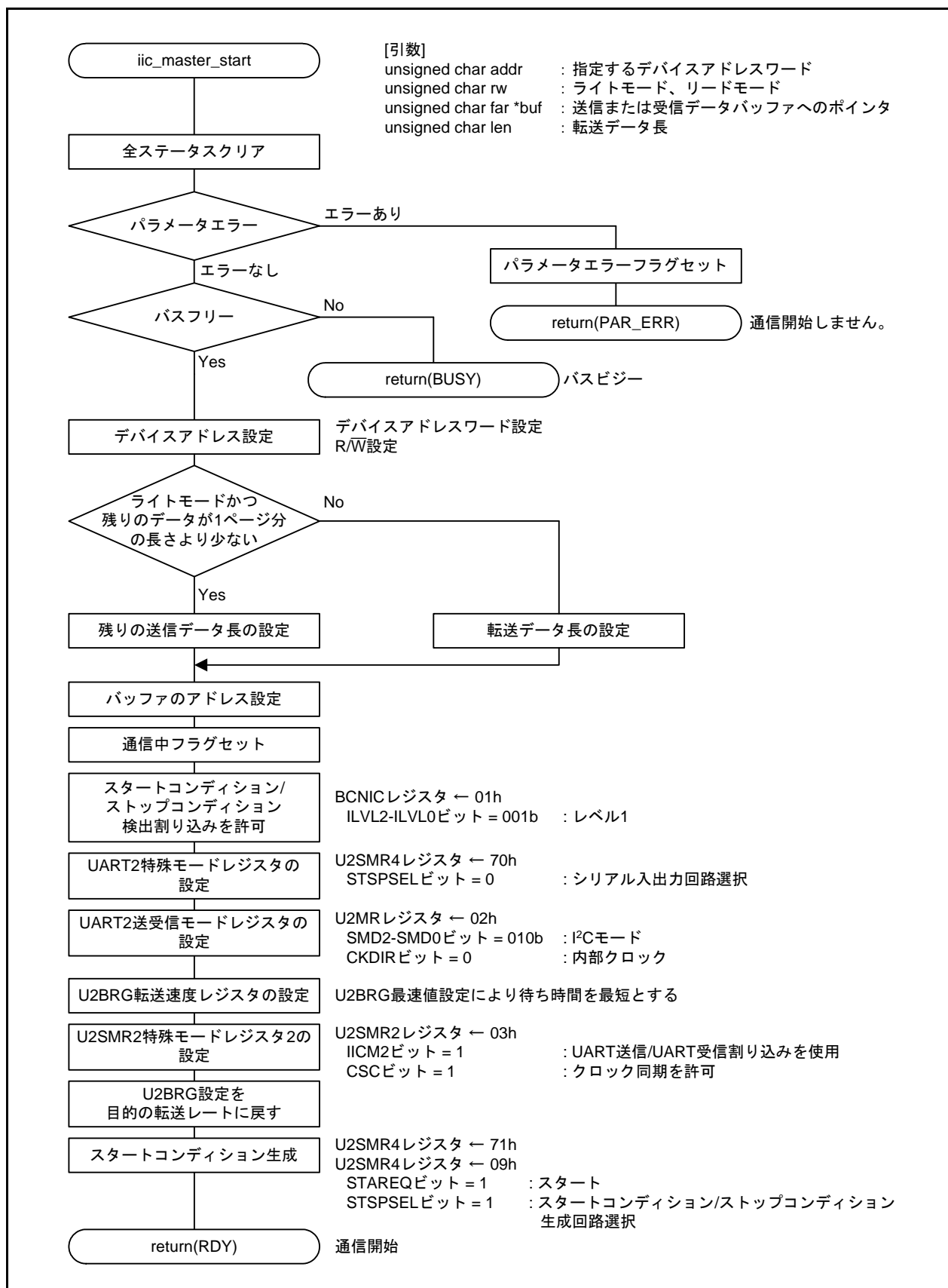
図 5.7 マスタ制御開始処理
