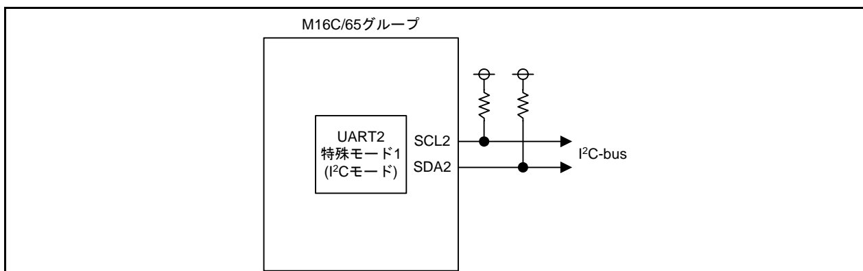
図 3.2 ブロック図
