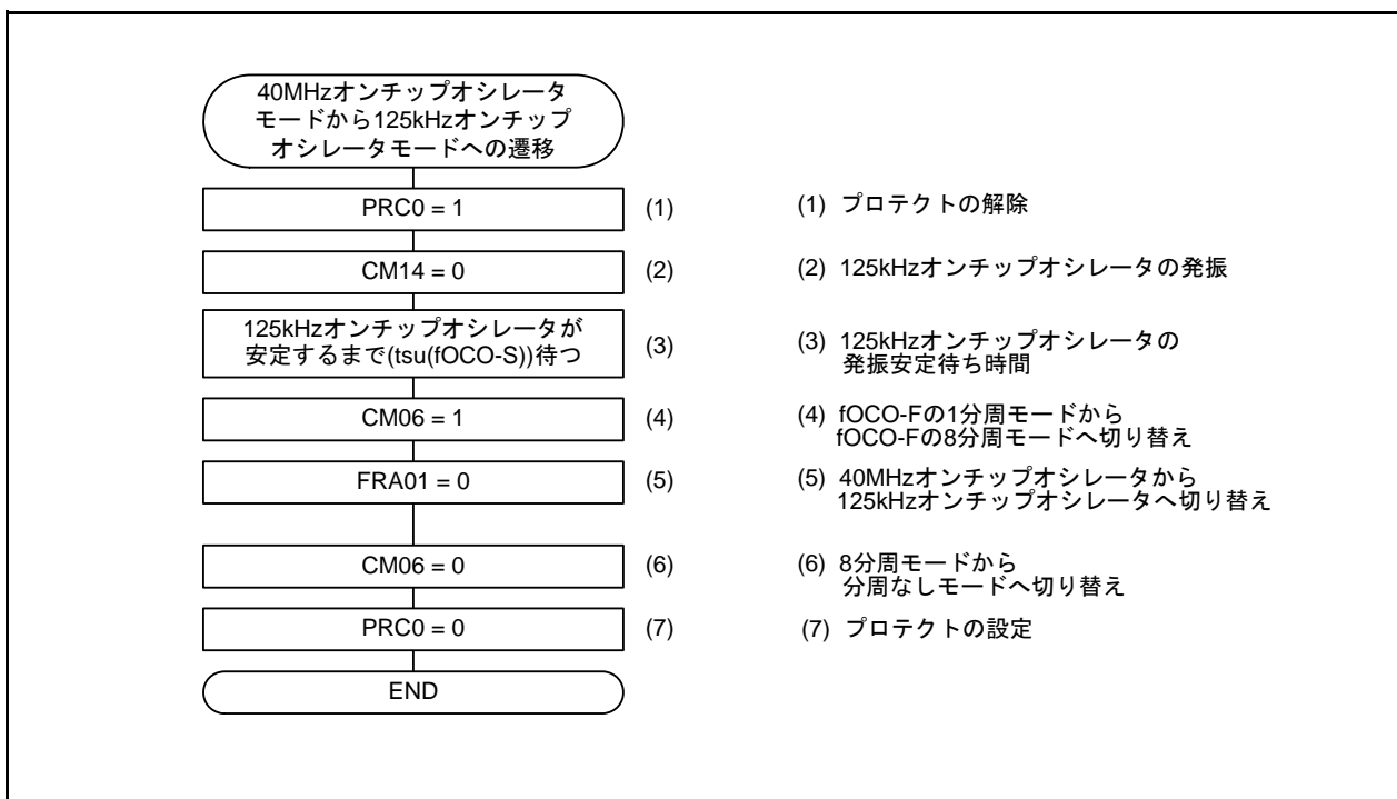
図3.2 40MHzオンチップオシレータモード(fOCO-Fの1分周)から125kHzオンチップオシレータモードへの遷移
