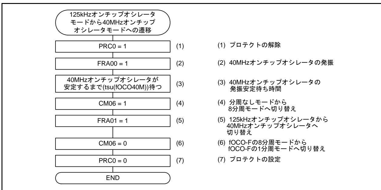
図3.5 125kHzオンチップオシレータモードから40MHzオンチップオシレータモード(fOCO-Fの1/4)への遷移
