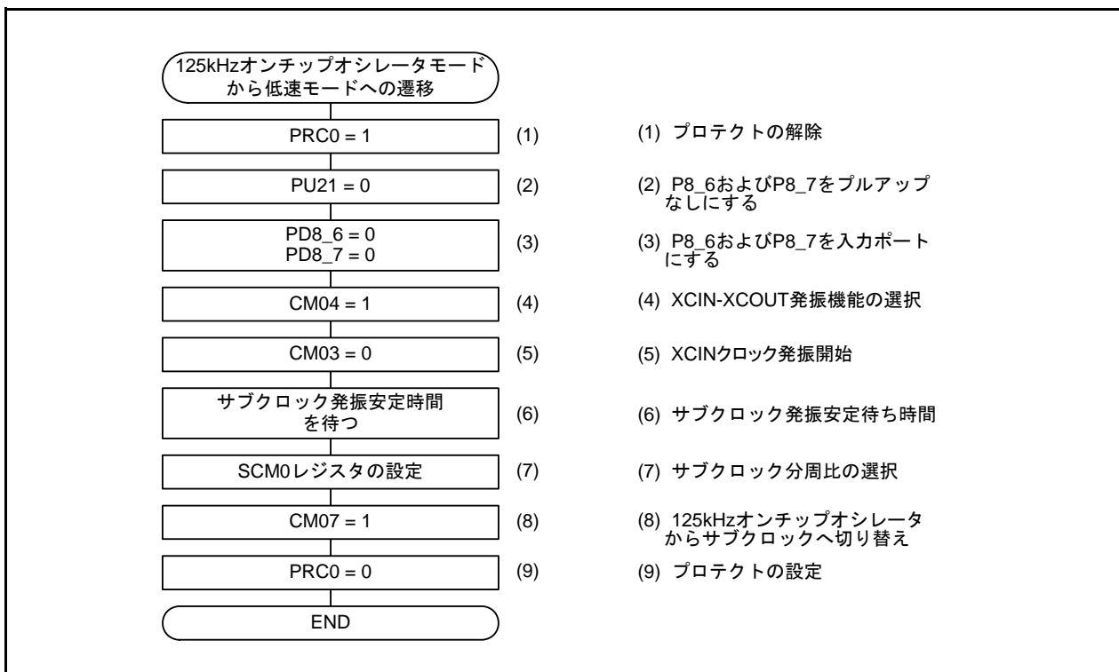
図 3.3 125kHzオンチップオシレータモードから低速モードへの遷移
