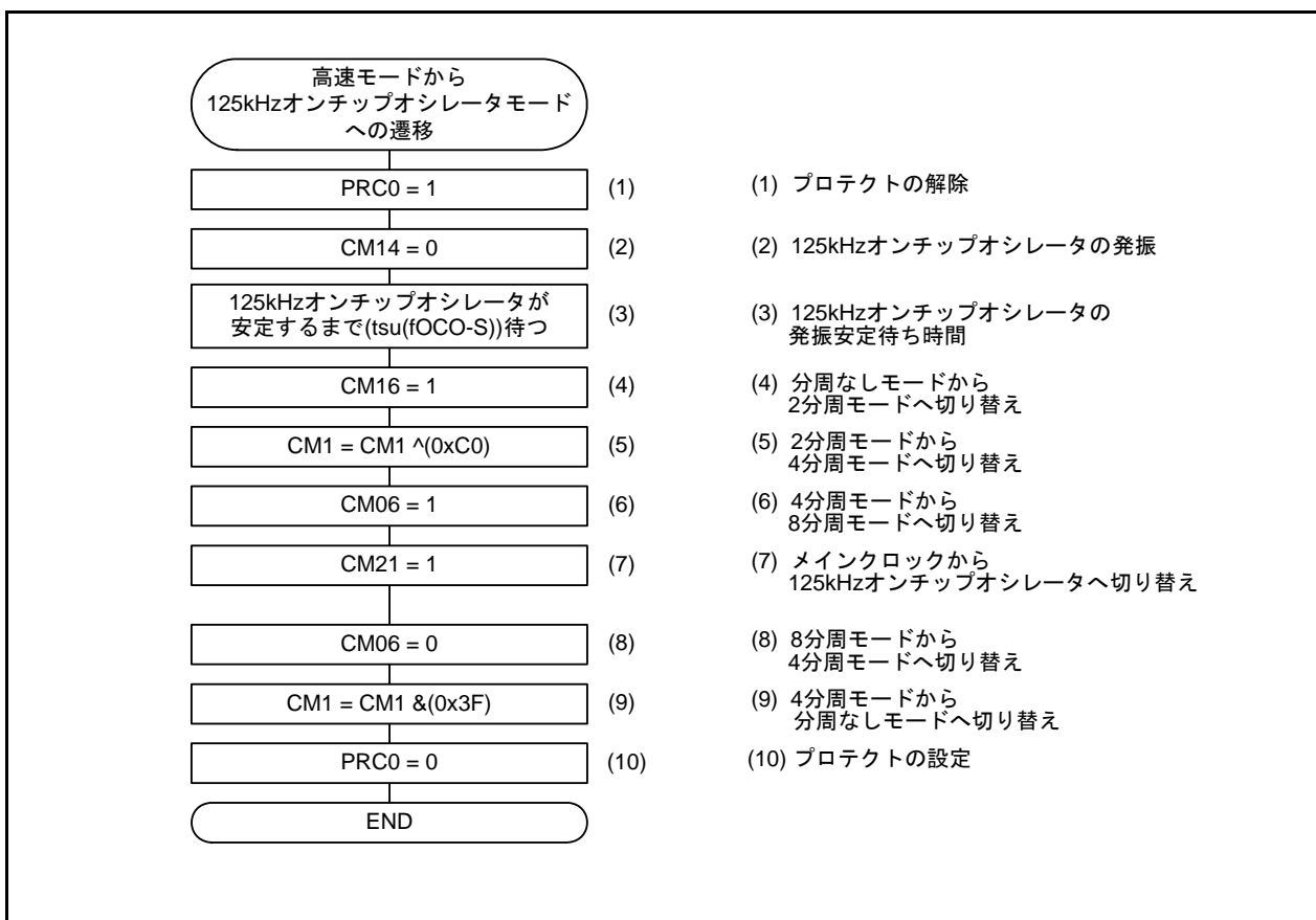
図3.2 高速モードから125kHzオンチップオシレータモードへの遷移
