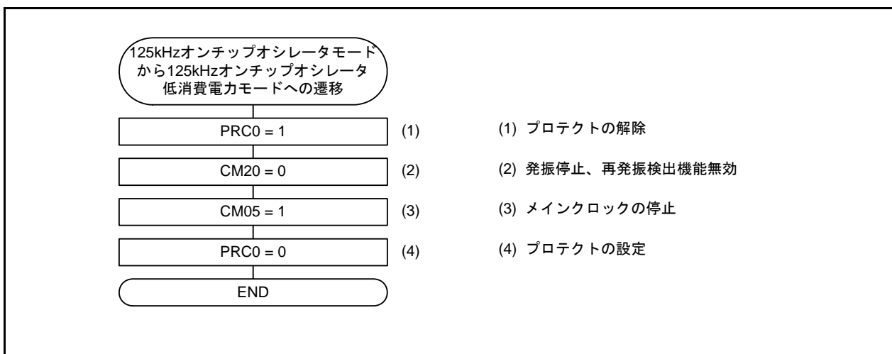
図3.3 125kHzオンチップオシレータモードから125kHzオンチップオシレータ低消費電力モードへの遷移
