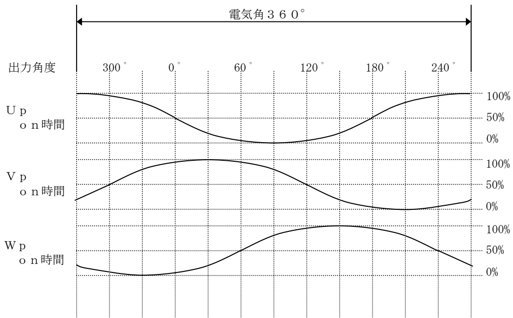
図 3.3.3 三相出力パターン
