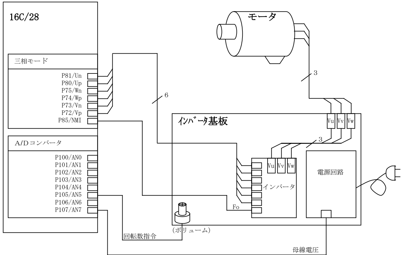
図 3.1.1 ハードウェア構成図
