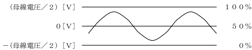
図 3.3.5 PWMデューティ
