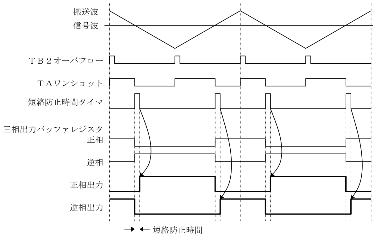
図 3.2.3 短絡防止時間
