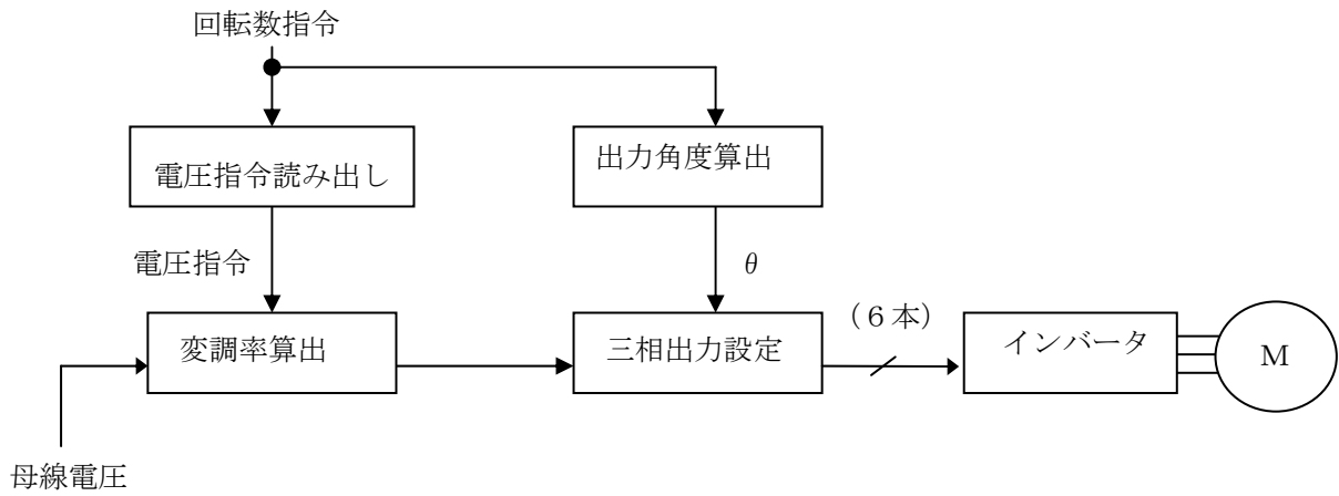
図 3.3.2 システム構成
