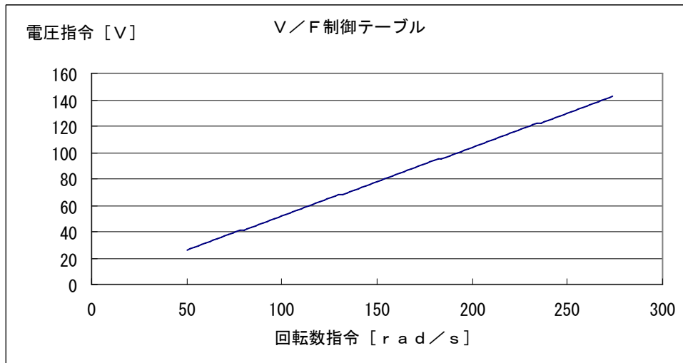
図 3.3.4 V/F制御テーブル
