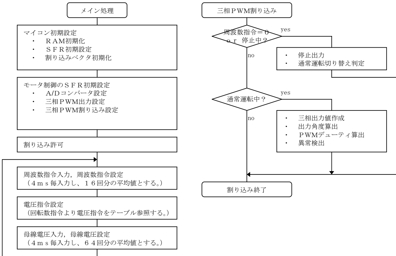
図 3.1.4 概略フロー図
