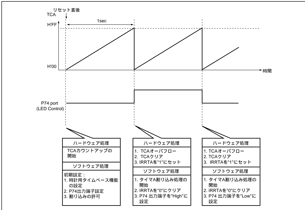
図 3.1 タイマ A 時計用タイムベース機能による LED 点滅動作の動作原理
