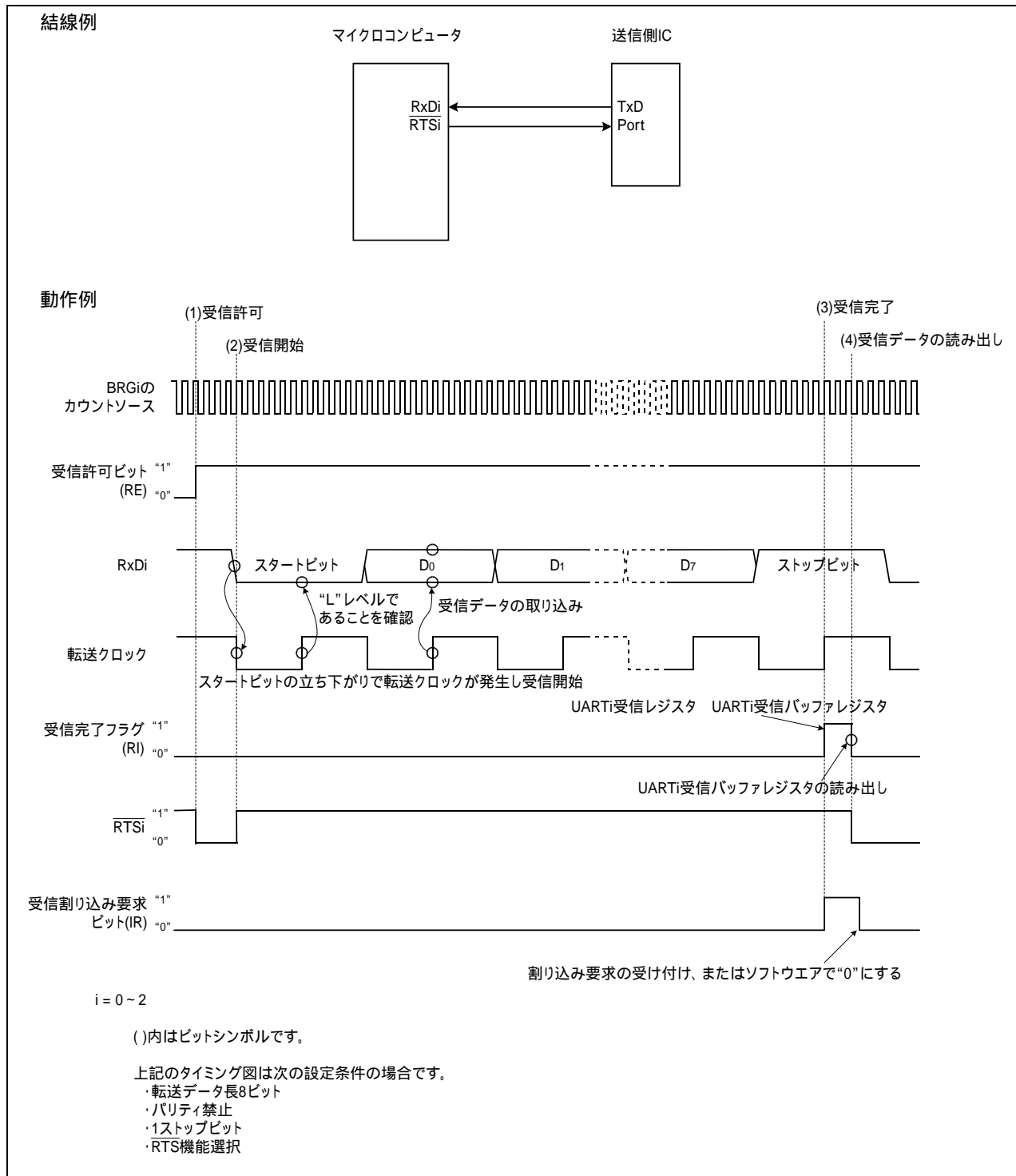
図 1 クロック非同期シリアル I/O モードの受信動作タイミング
