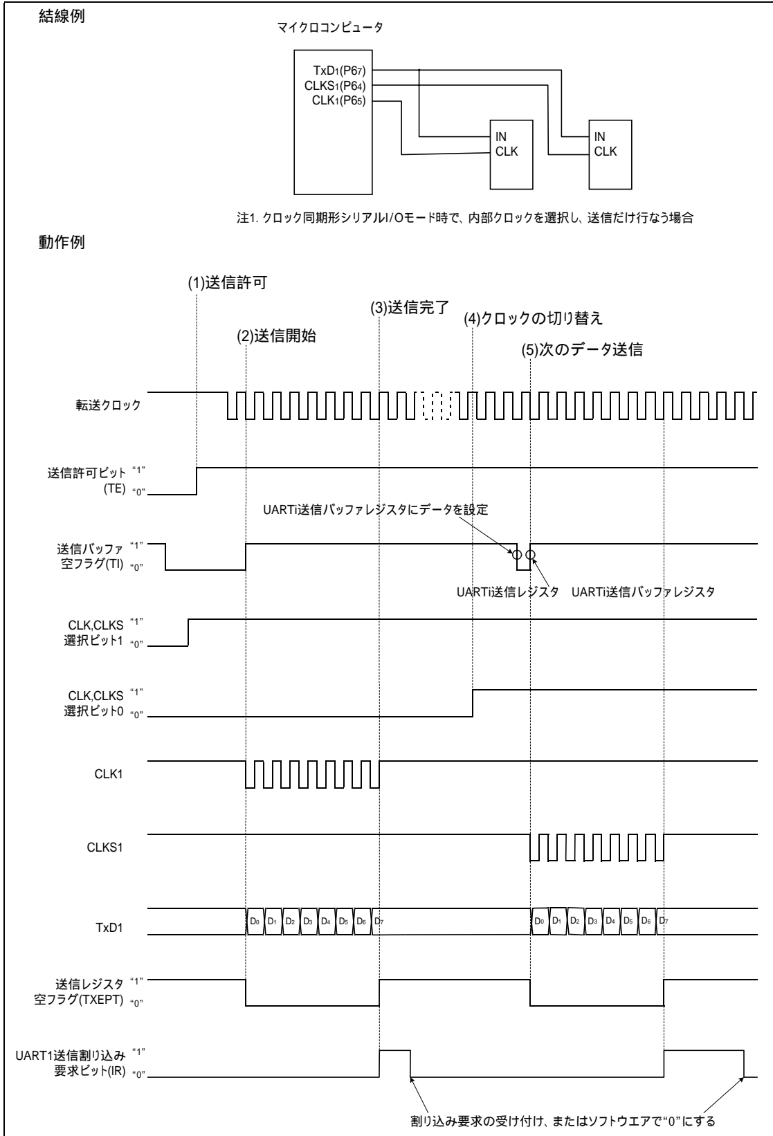
図 1 クロック同期形シリアル I/O モードの送信、複数クロック出力機能選択時の動作タイミング
