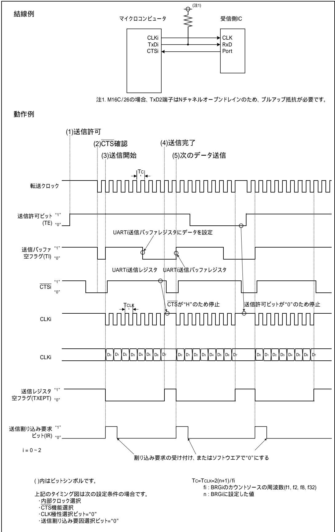
図 1 クロック同期形シリアル I/O モードの送信動作タイミング
