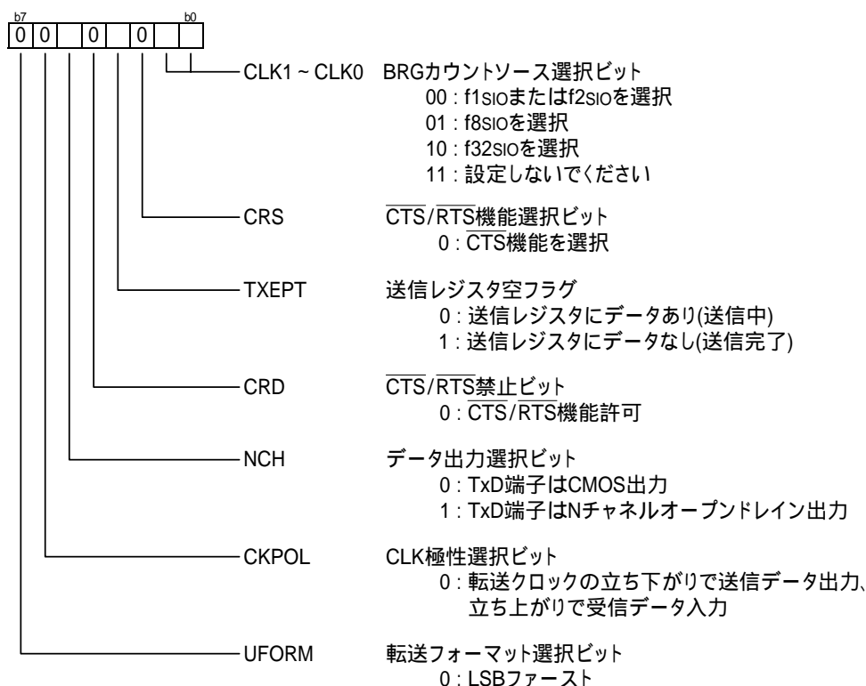
(2) UARTi送受信制御レジスタ0の設定(i=0,1)
