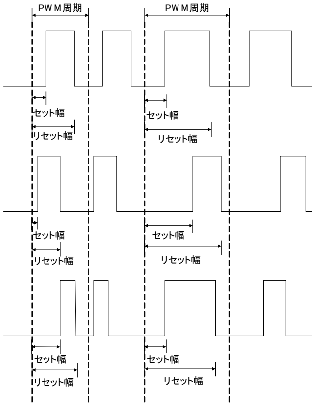
PWM出力波形
