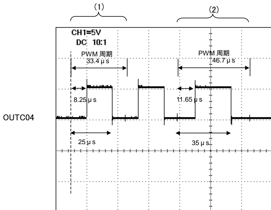
オシロスコープによる測定結果
