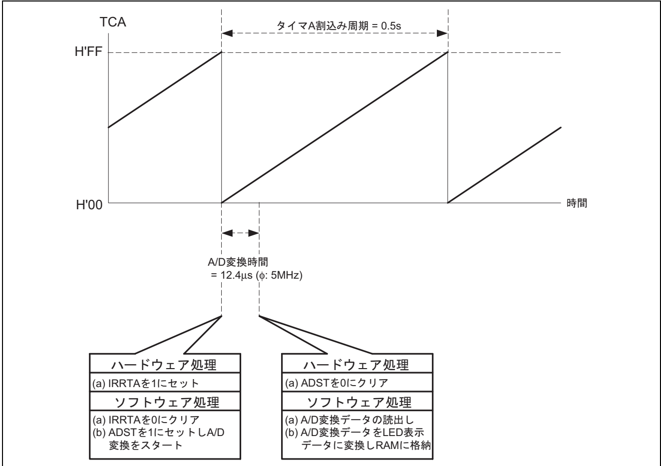
図 6 タイマ A を使用した AN0 端子の A/D 変換の動作原理
