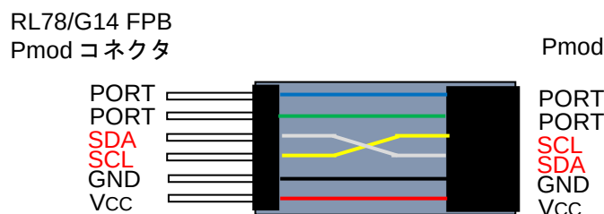
図 1.1 信号変換
