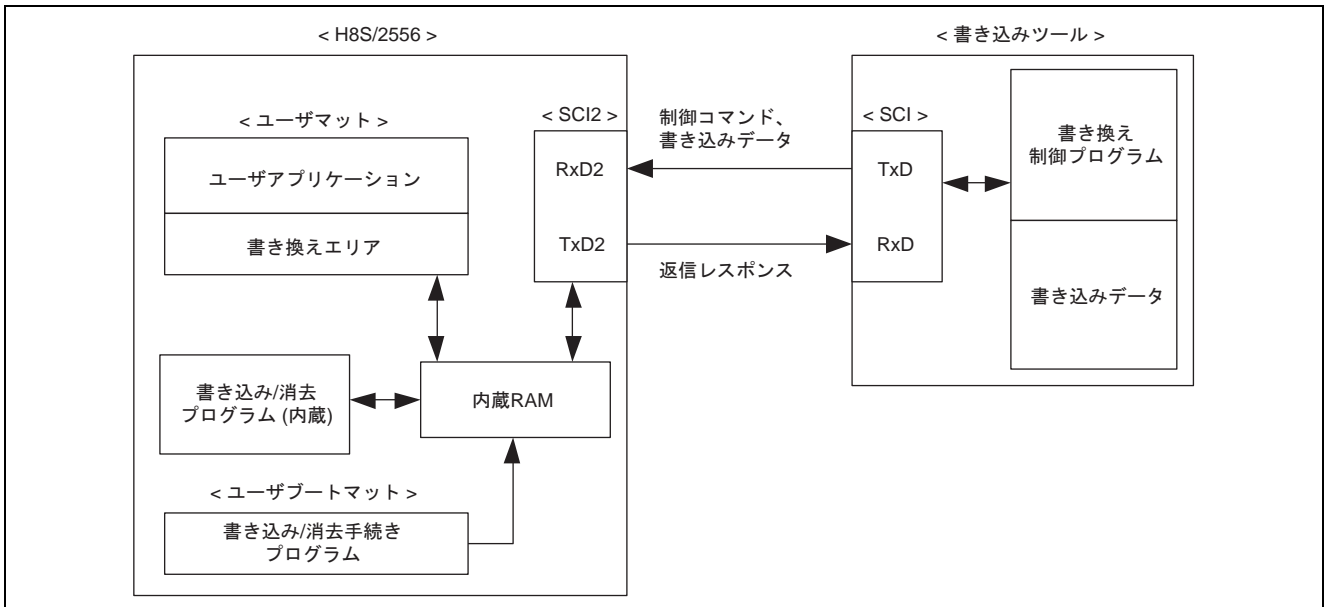
図 1 SCI (調歩同期式) を使用したオンボード書き換え構成図
