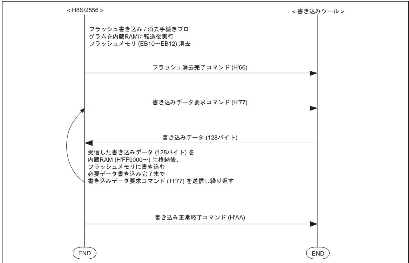
図 2 制御コマンド動作
