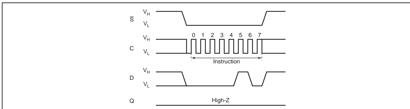
図 4 WREN 動作
