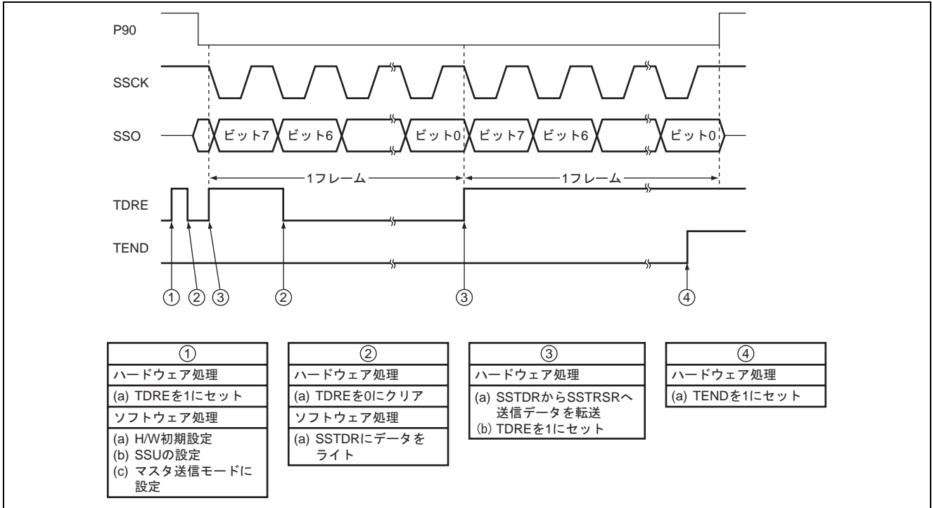
図8 送信モード動作タイミング
