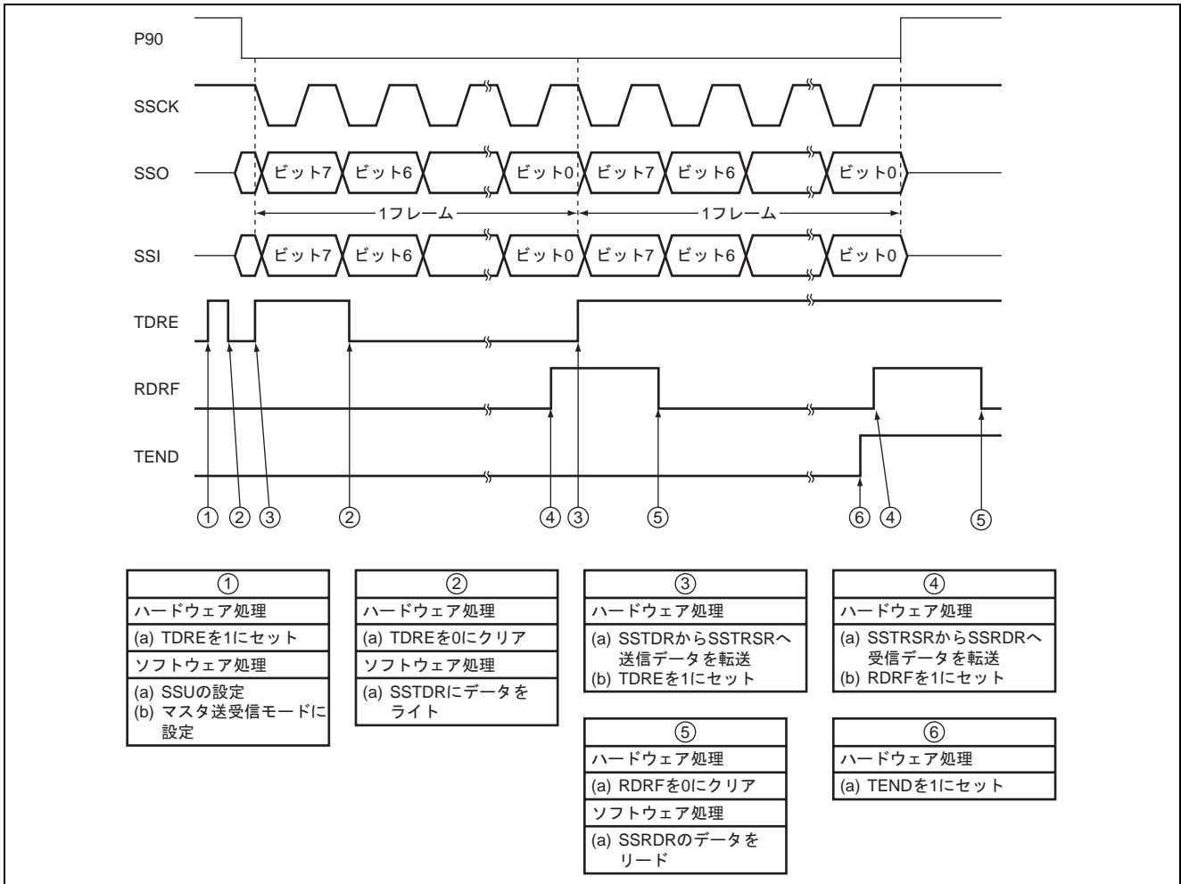
図9 送受信モード動作タイミング
