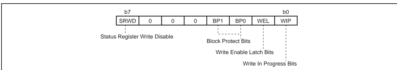
図 3 EEPROM ステータスレジスタ構成図
