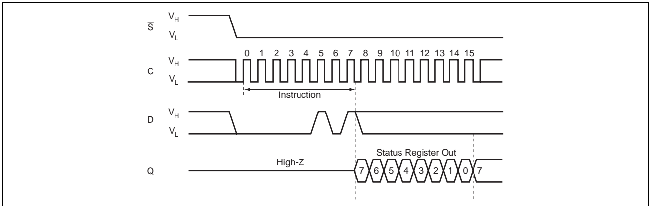
図 5 RDSR 動作
