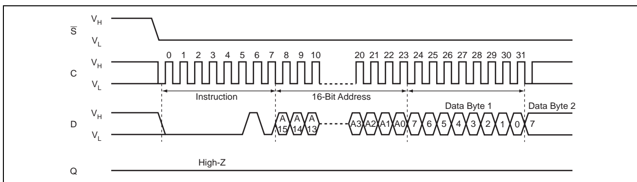
図7 WRITE 動作
