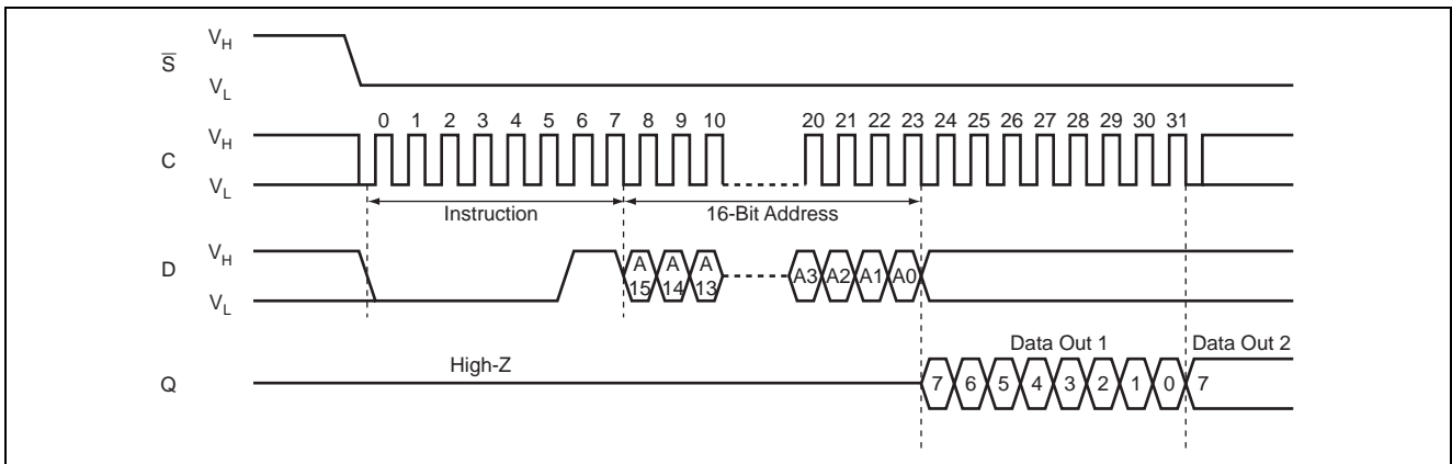
図 6 READ 動作
