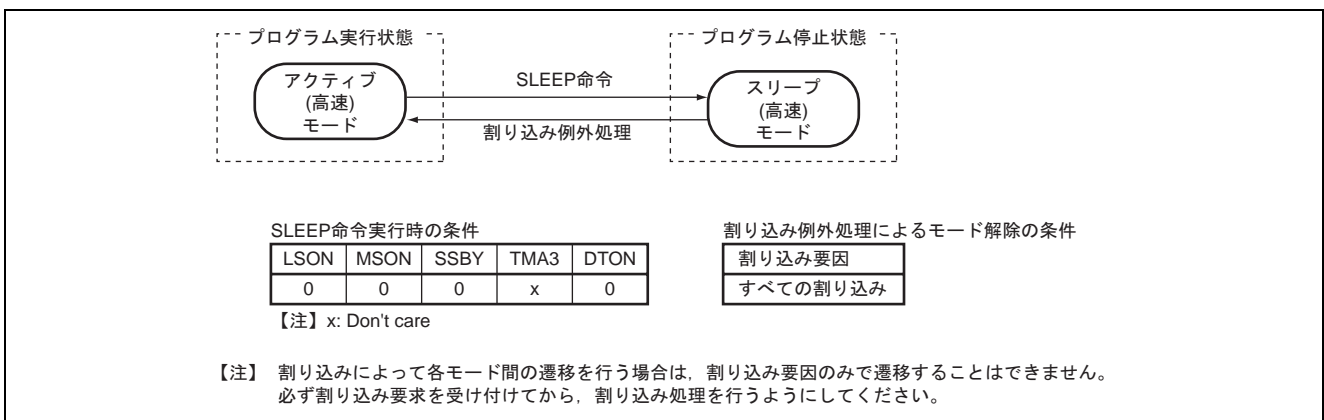
図1 モード遷移図
