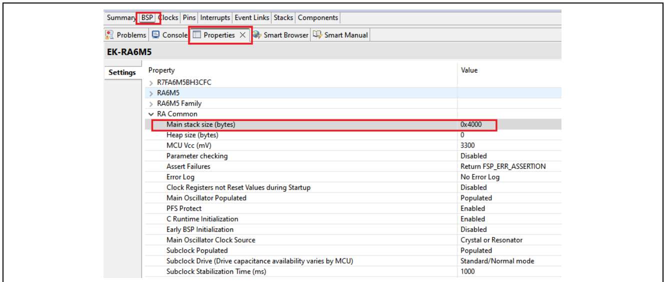
图 20. 更改 Main Stacks Size
