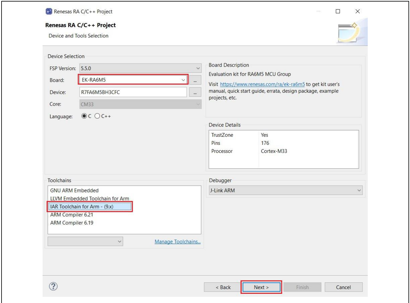
图 12. RA 工程选项
