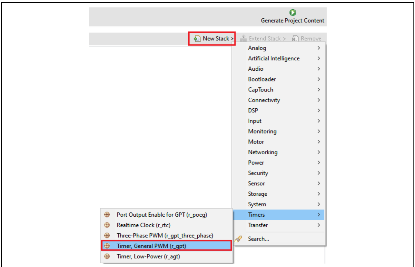
图 18. 添加 GPT 定时器
