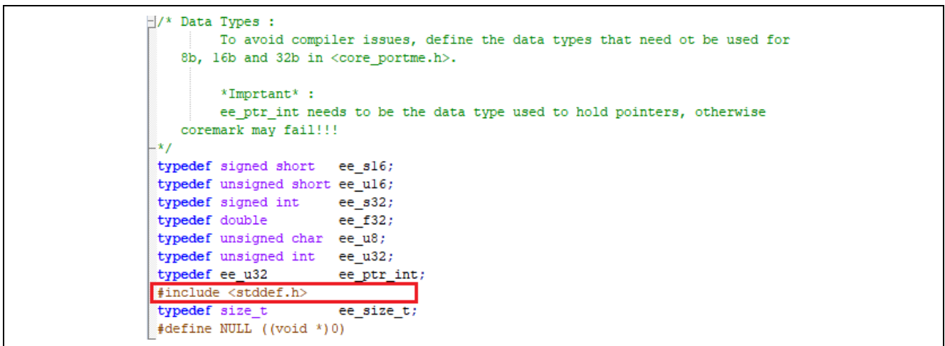
图 22. 添加 “#include <stddef.h>”
