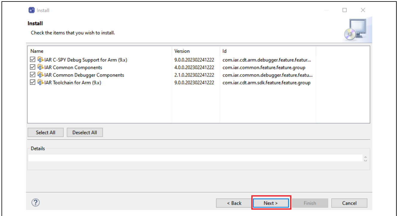
图 4. 安装 IAR Embedded Workbench 插件
