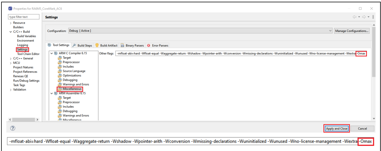
图 35. 在工程设置中添加 “ -Omax ” 选项
