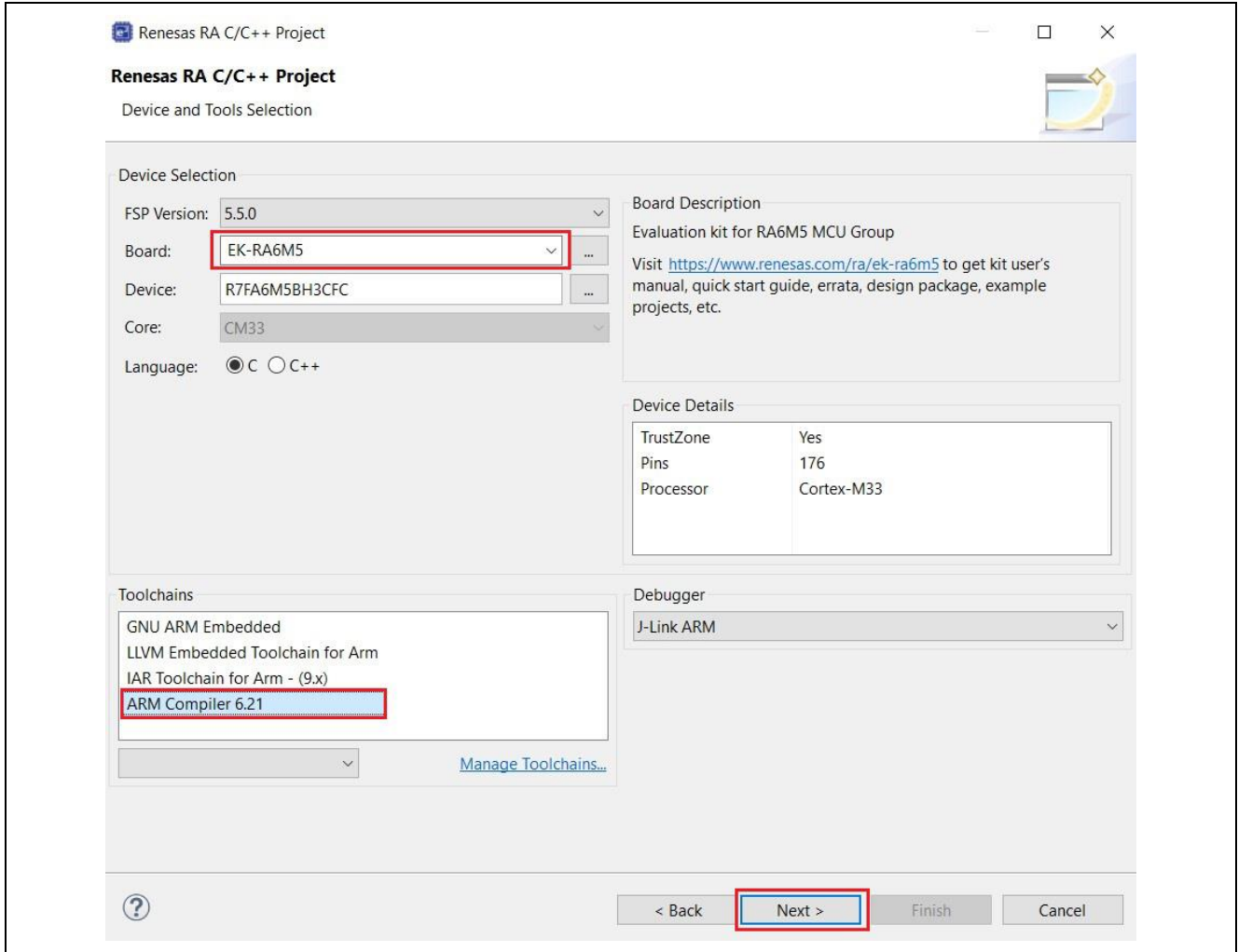
图 33. 创建基于 Arm Compiler 的工程选项
