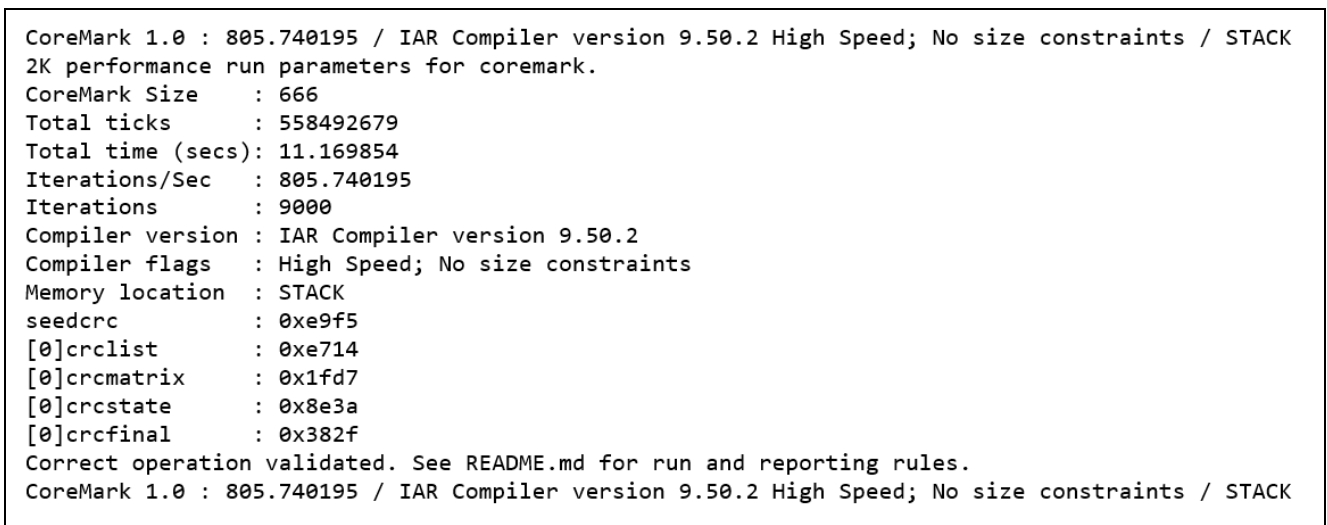
图 42. 通过 IAR Compiler 进行 CoreMark 评分
