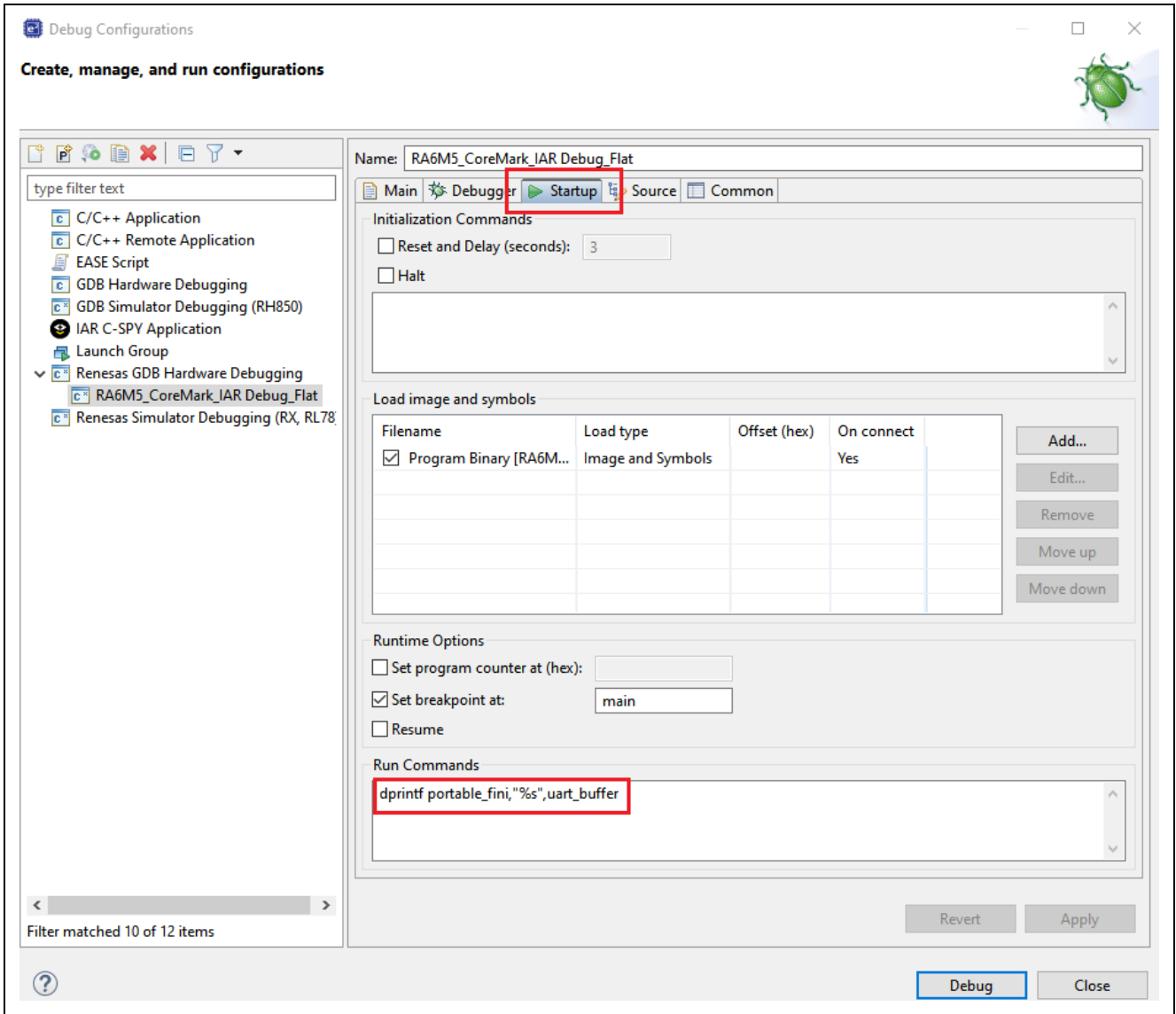
图 39. 添加 dprintf 指令
