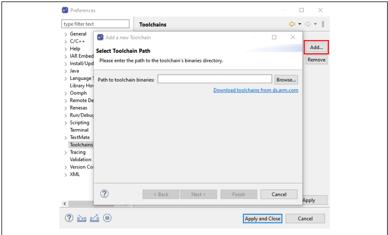
图 9. 添加 Toolchains 的路径
