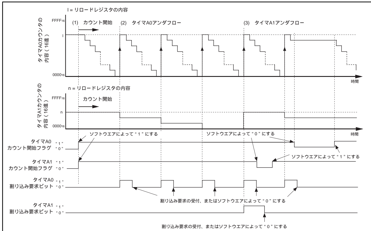
図1 長い周期のタイマの動作タイミング
