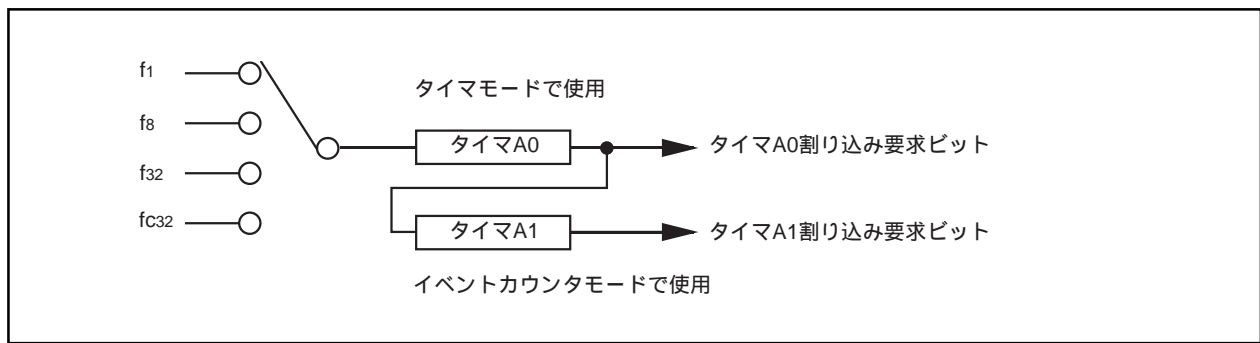
図2 長い周期のタイマのタイマ接続図
