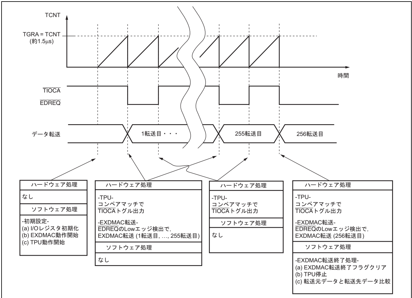
図 7 動作説明図
