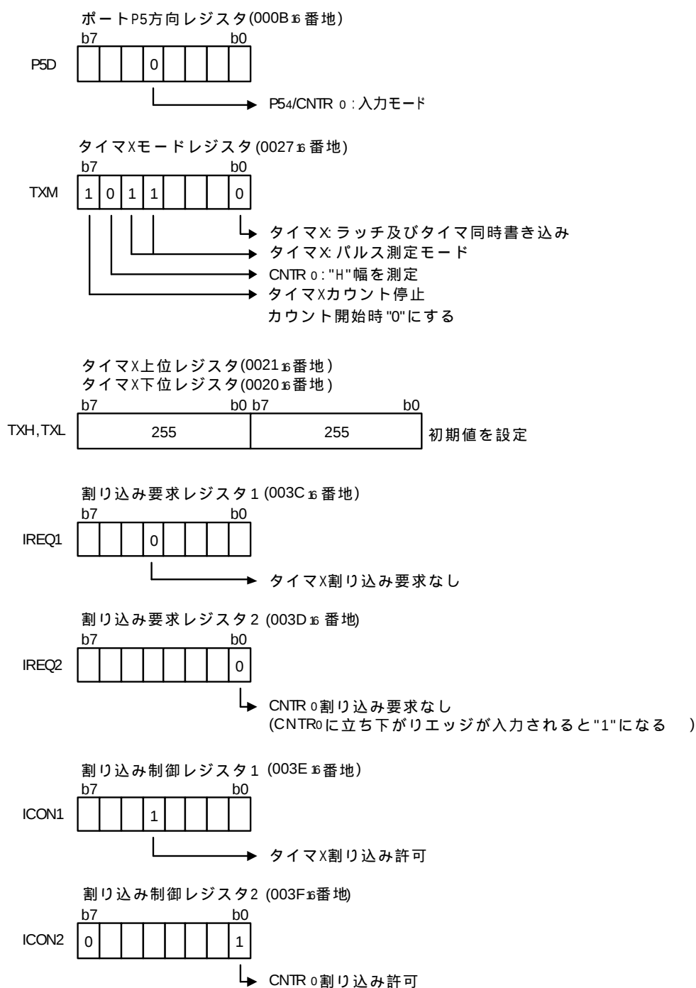
図 3.2 関連レジスタの設定
