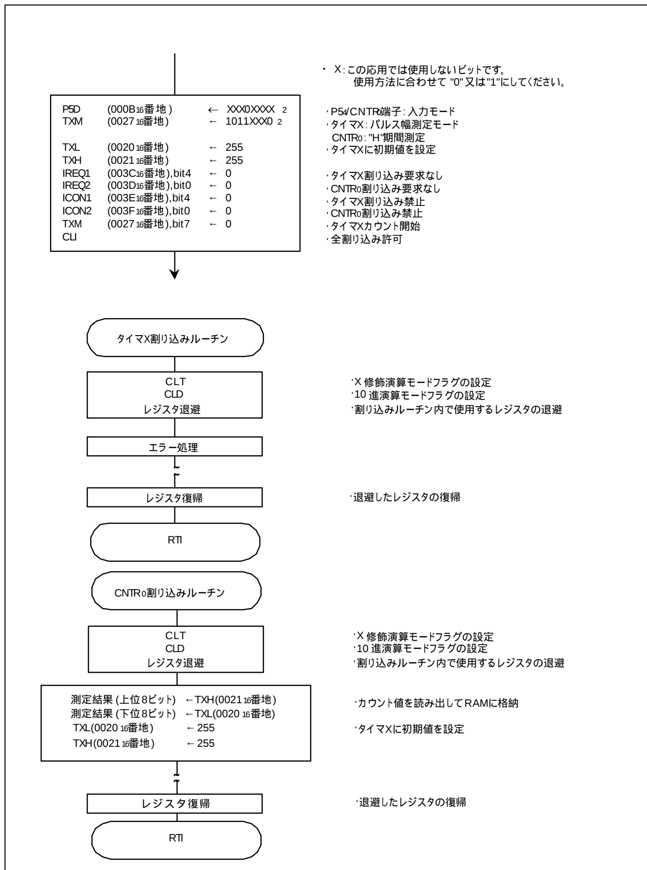
図 3.3 制御手順
