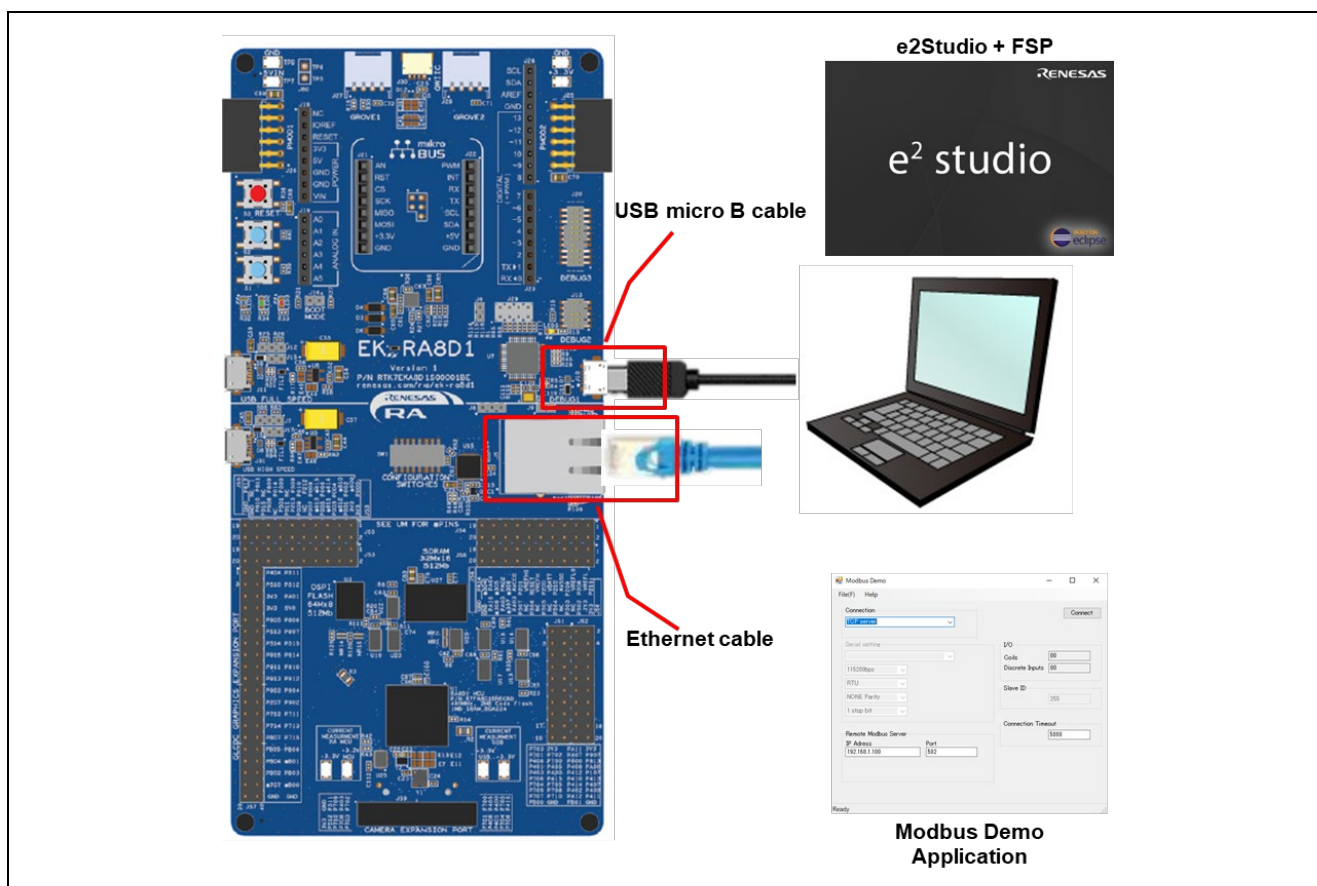
図 5: EK-RA8D1 board 接続設定
