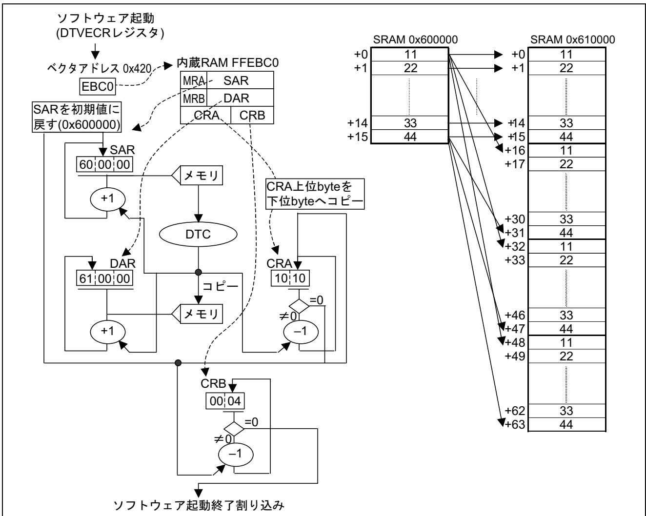
図 4 ブロック転送モード動作フロー
