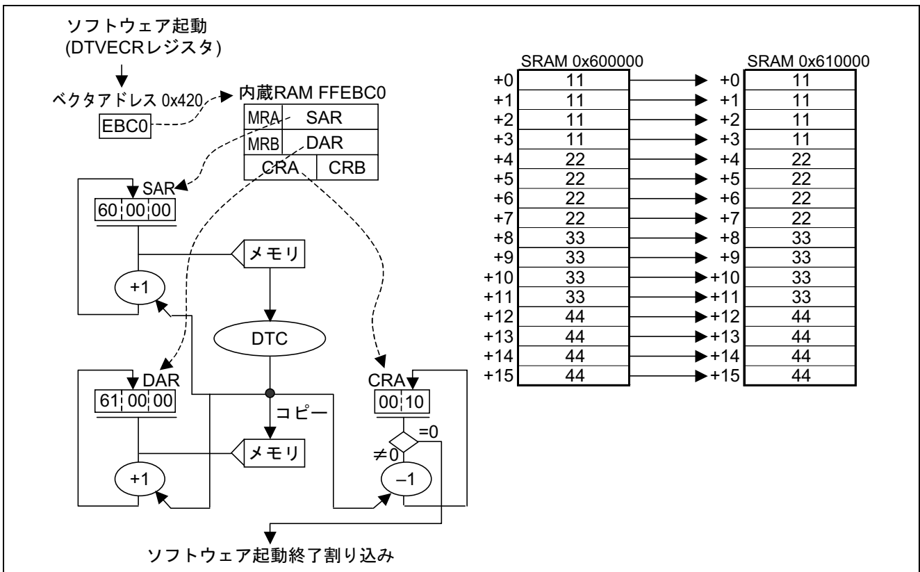
図2 ノーマルモード動作フロー
