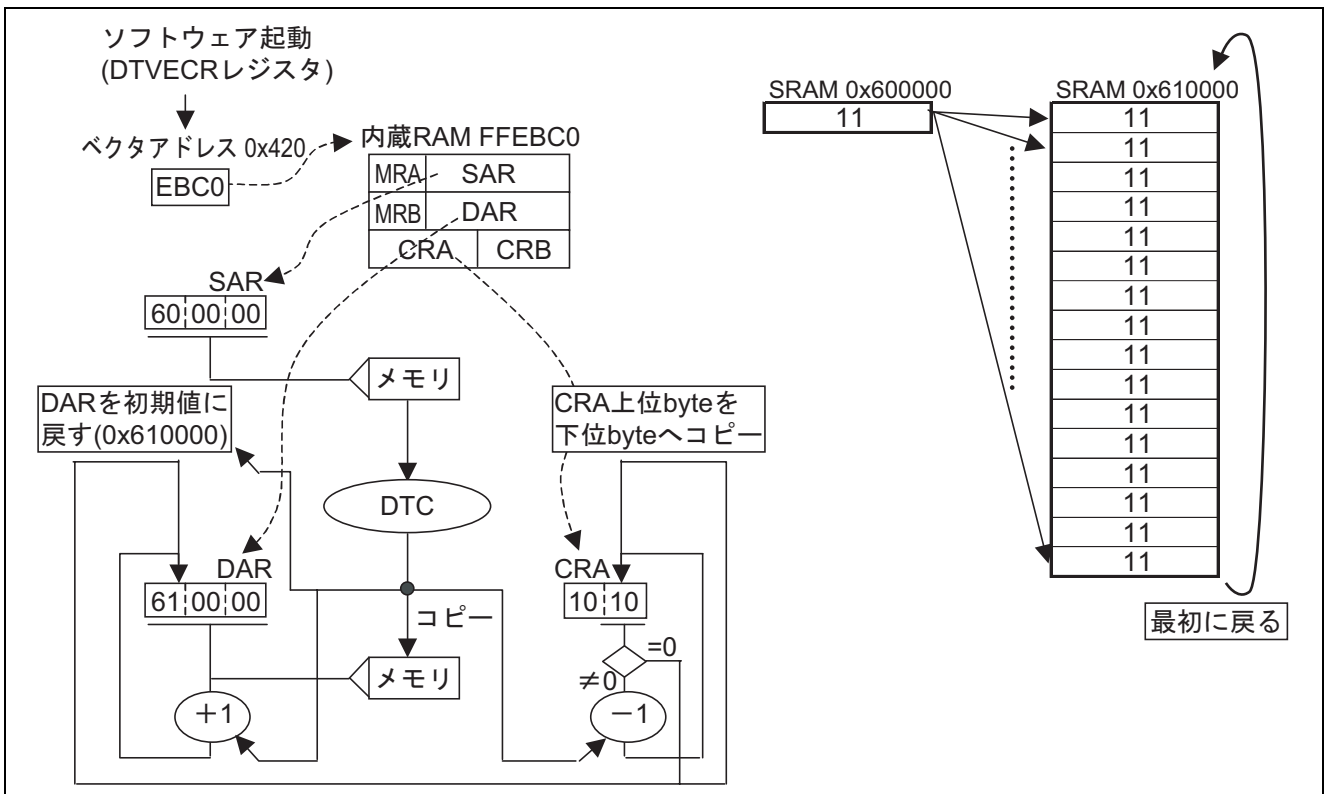
図3 リpeatモード動作フロー
