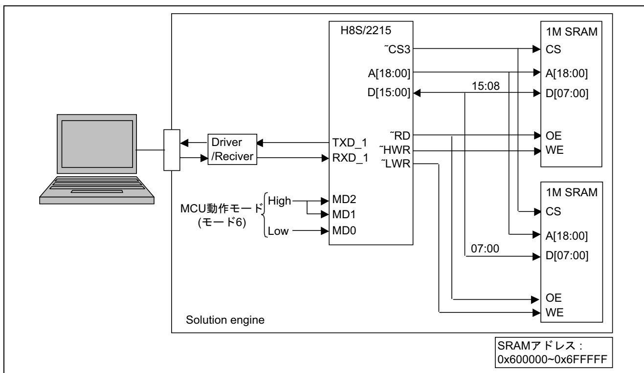
図 1 確認構成
