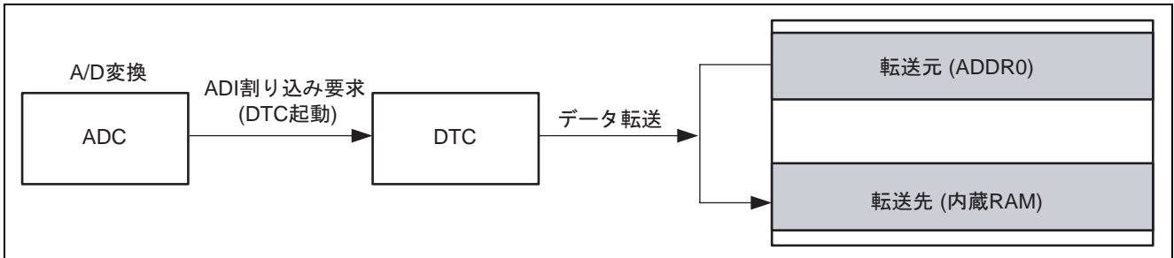
図 1 DTC 動作概要
