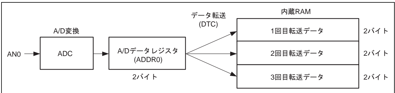
図 2 ノーマル転送モードでのデータの流れ
