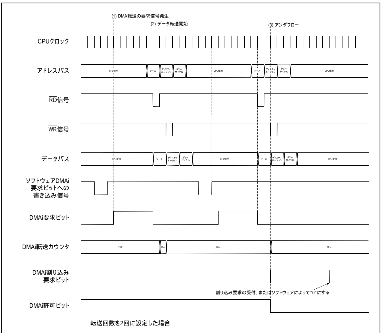
図 1 単転送モードの動作例
