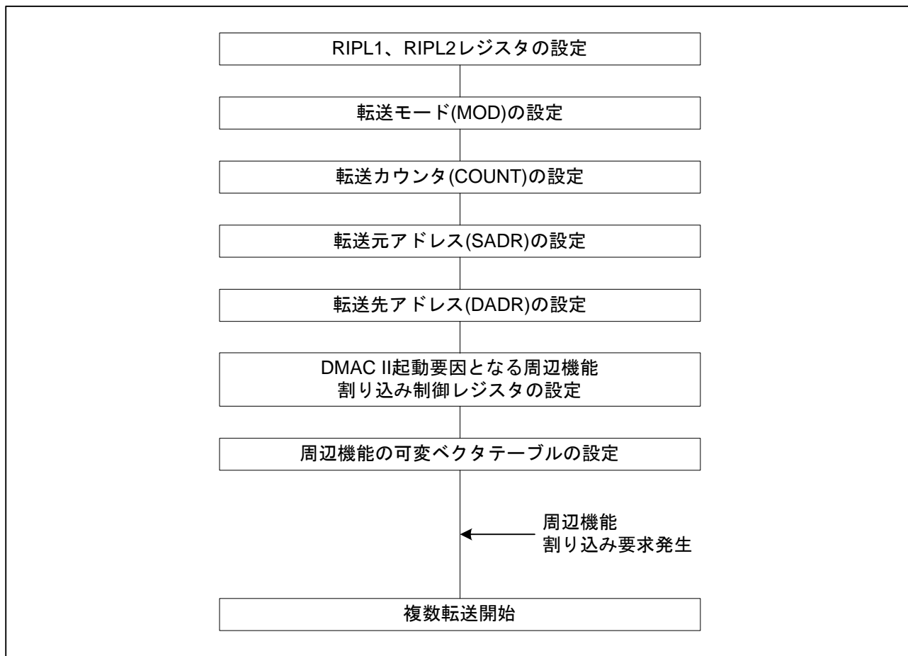
図4. DMAC IIでの複数転送の設定手順
