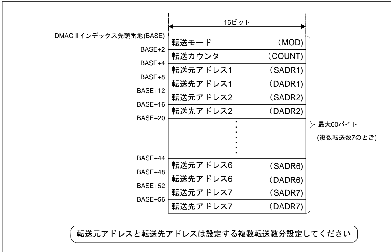
図2. 複数転送でのDMAC IIインデックス
