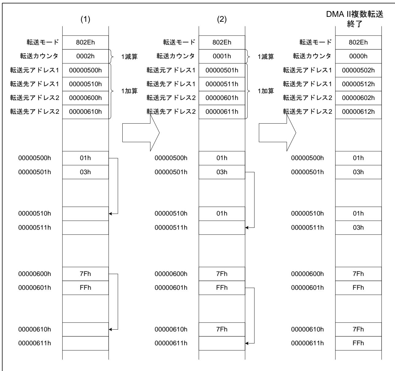
図1. 本アプリケーションノートの設定によるDMAC IIの複数転送動作イメージ図
