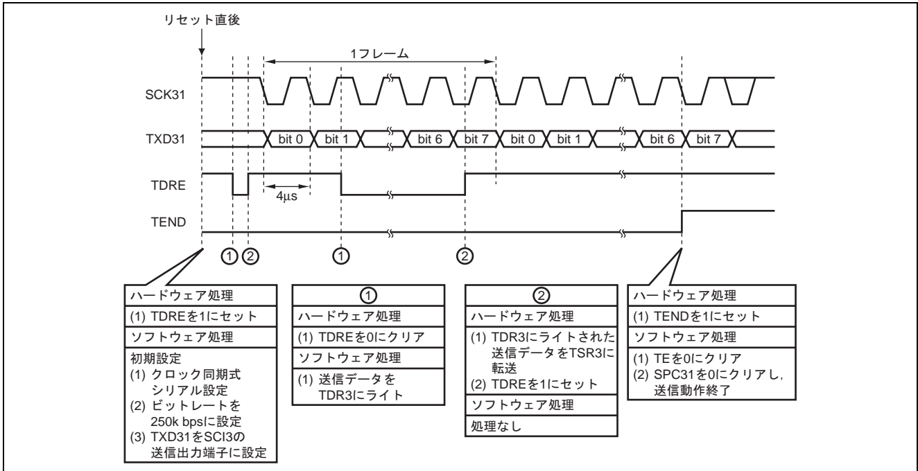
図3 クロック同期式モードのシリアルデータ送信の動作説明
