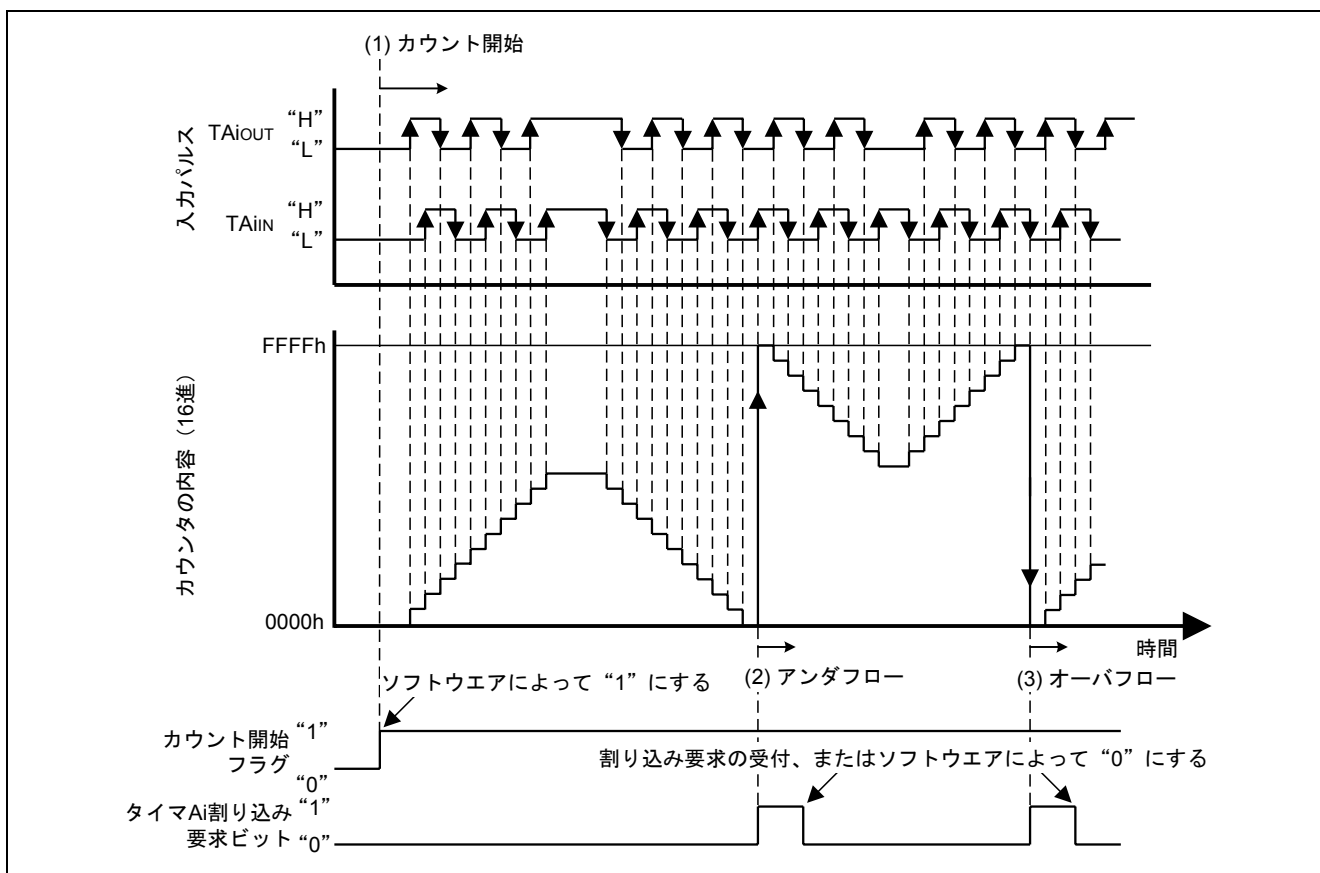
図 1. イベントカウンタモード二相パルス信号処理、4 逓倍処理動作時の動作タイミング
