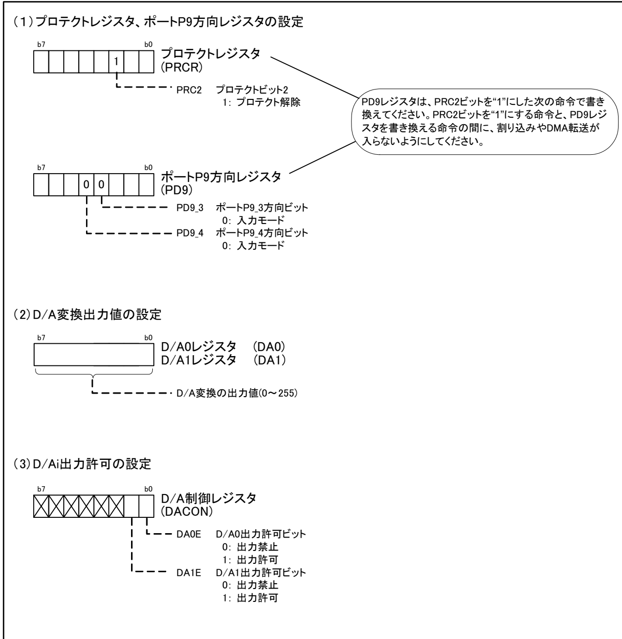
図 4.1 D/A コンバータのレジスタ設定
