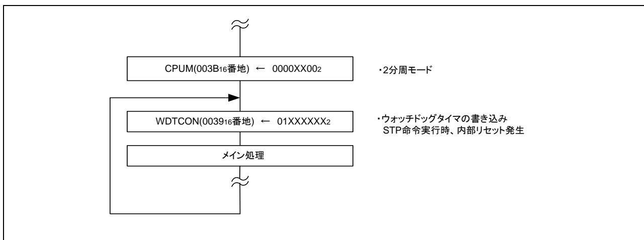
図 3.3 制御手順
