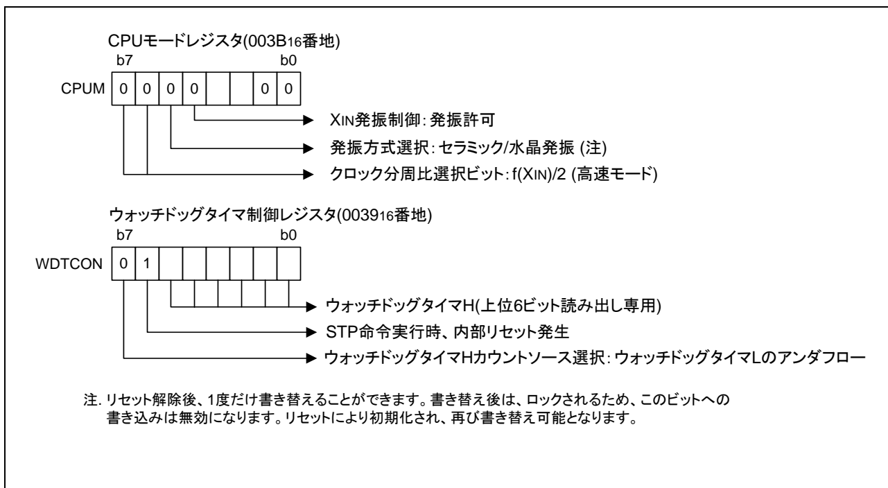
図 3.2 関連レジスタの設定
