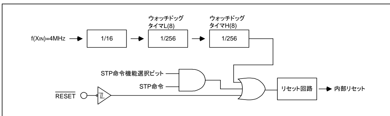
図 3.1 接続と分周比の設定
