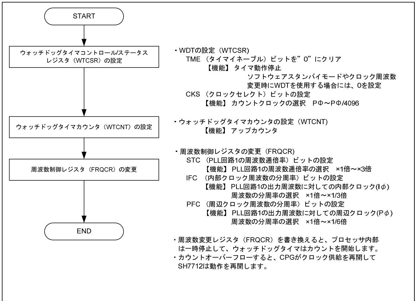
図3 動作周波数変更のための設定フロー例
