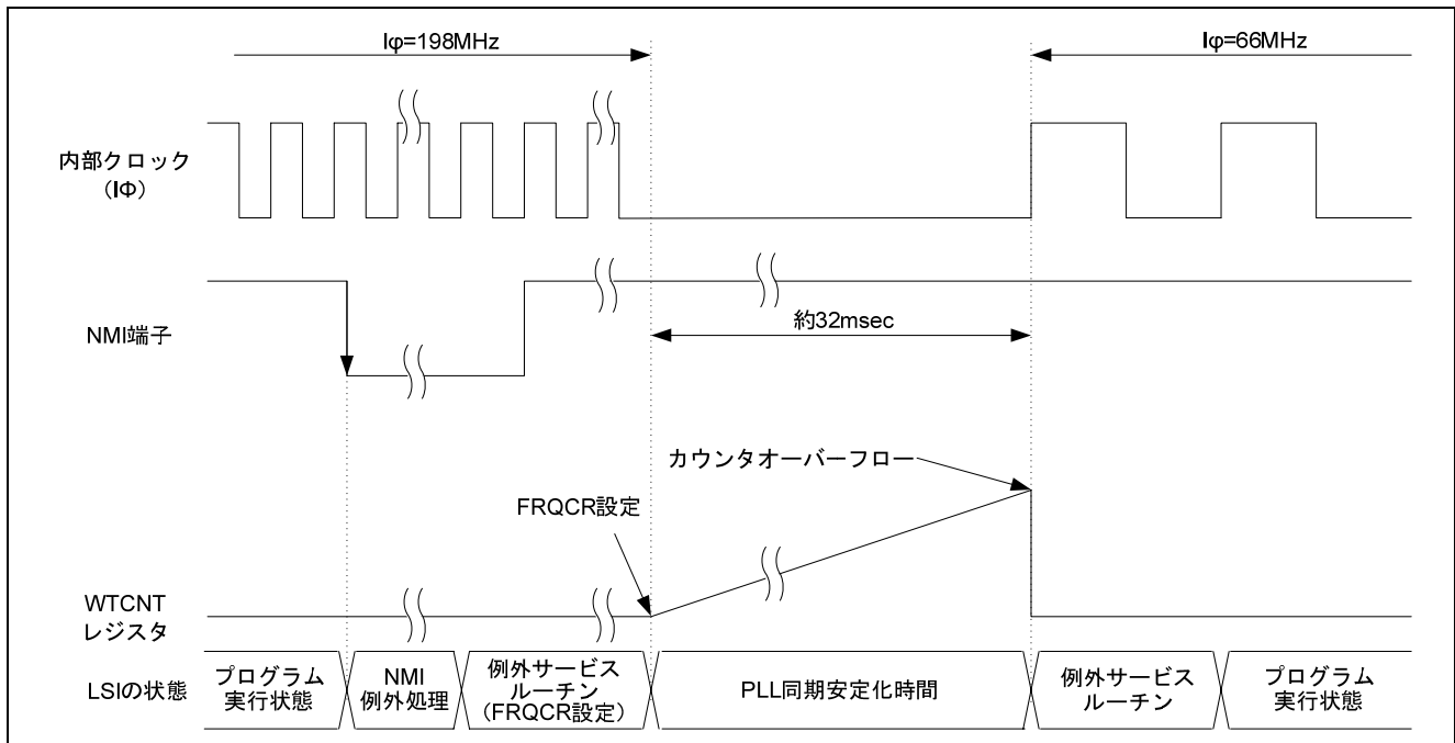
図4 参考プログラムの動作タイミングイメージ図
