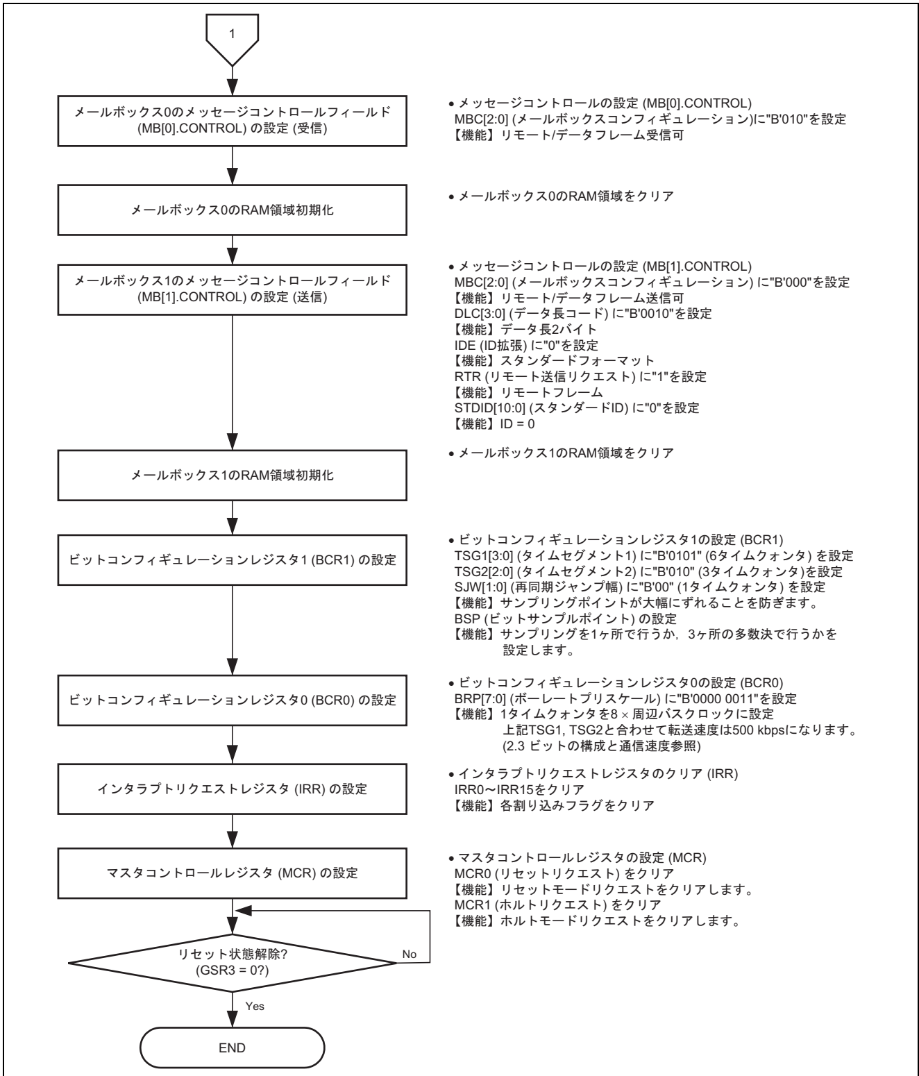
図 3 RCAN-ET の初期設定フロー例 (2)
