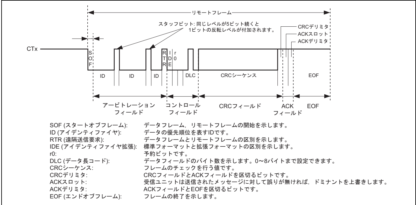
図 5 リモートフレームの送信波形
