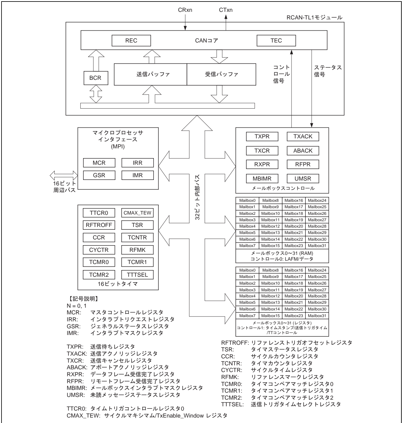
図 1 RCAN-TL1 の構成図
