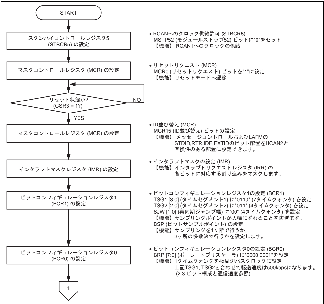
図 2 RCAN-TL1 の初期設定フロー例 (1)
