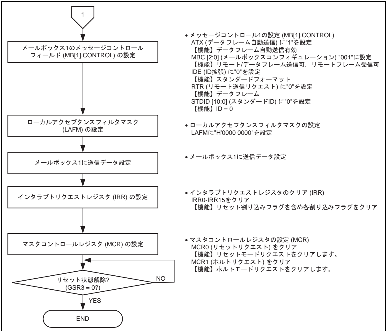
図3 RCAN-TL1の初期設定フロー例 (2)
