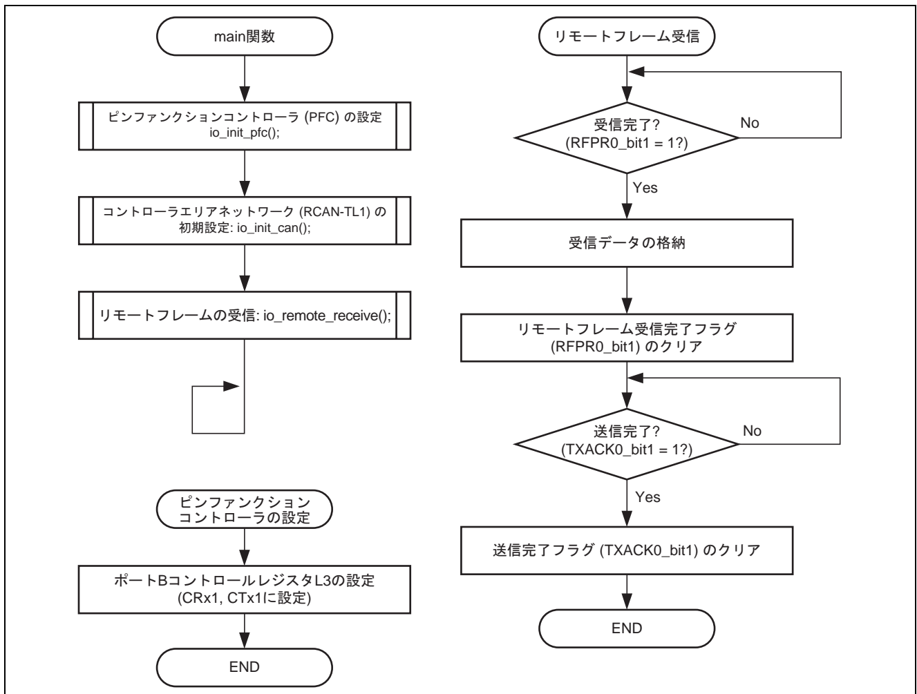
図6 参考プログラムの処理フロー例
