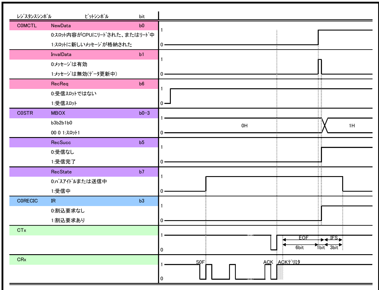
図1 CAN 受信時の各フラグの動作タイミング
