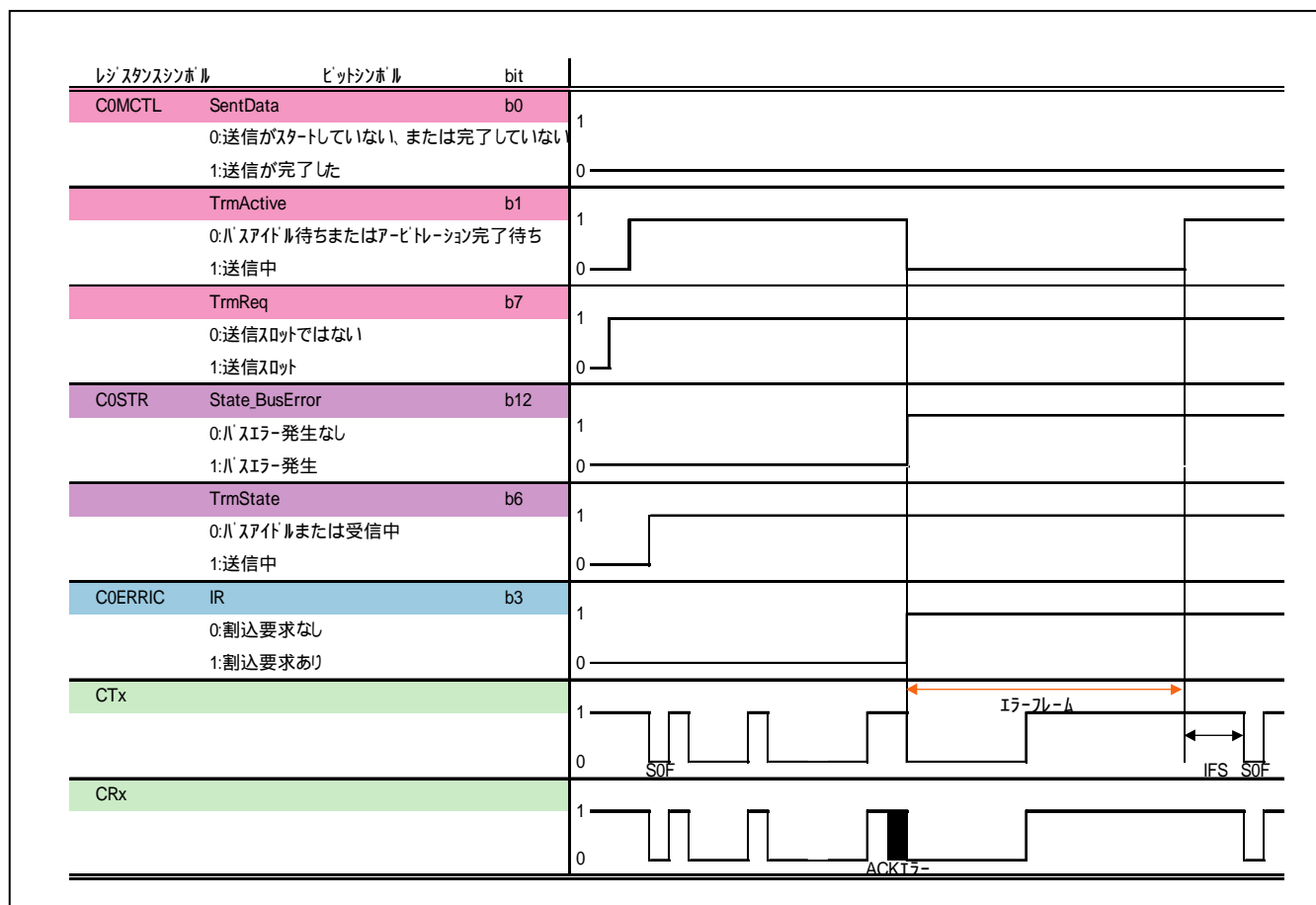
図 1. CAN エラー発生時の各フラグ動作
