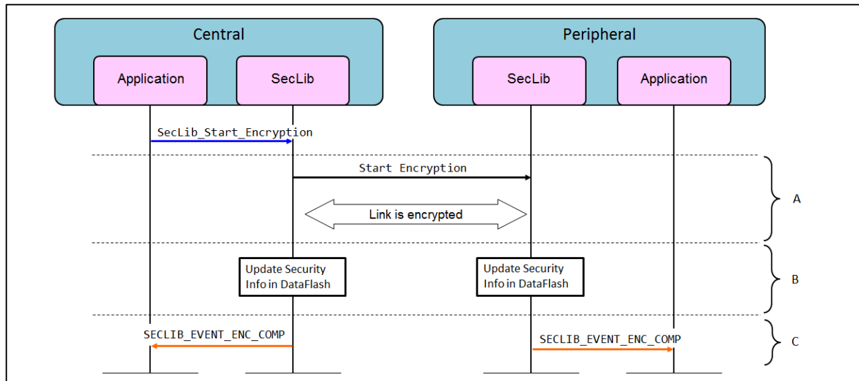
図 2-8 暗号化の動作シーケンス
