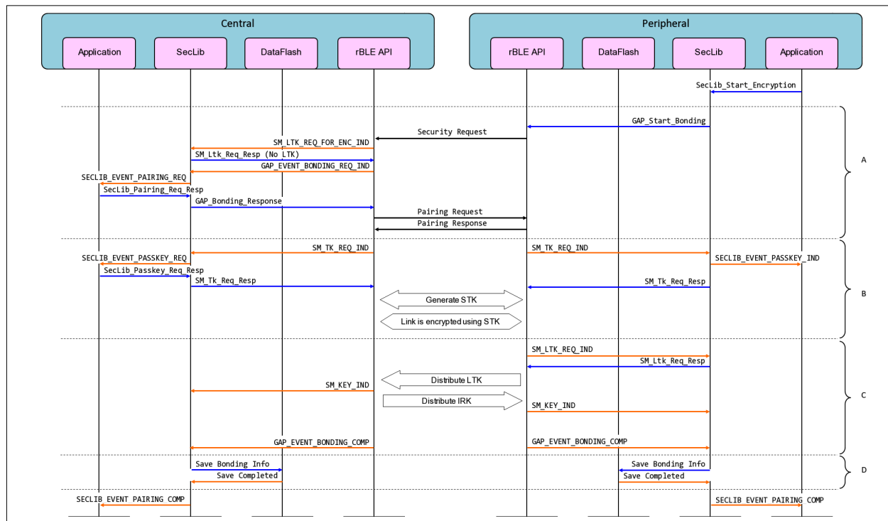
図 5-4 Peripheral 開始ペアリングシーケンス
