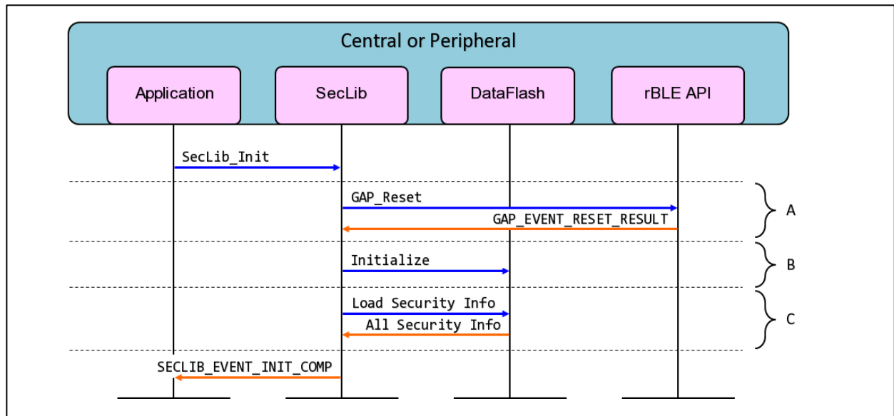
図 5-1 初期化シーケンス
