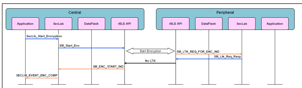
図 6-2 脆弱性を回避するシーケンス
