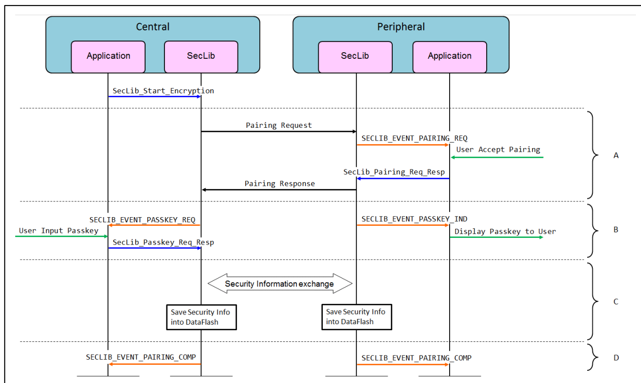
図 2-3 ペアリングの動作シーケンス
