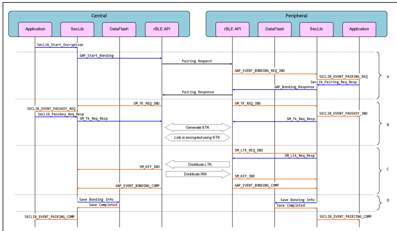
図 5-3 Central 開始ペアリングシーケンス
