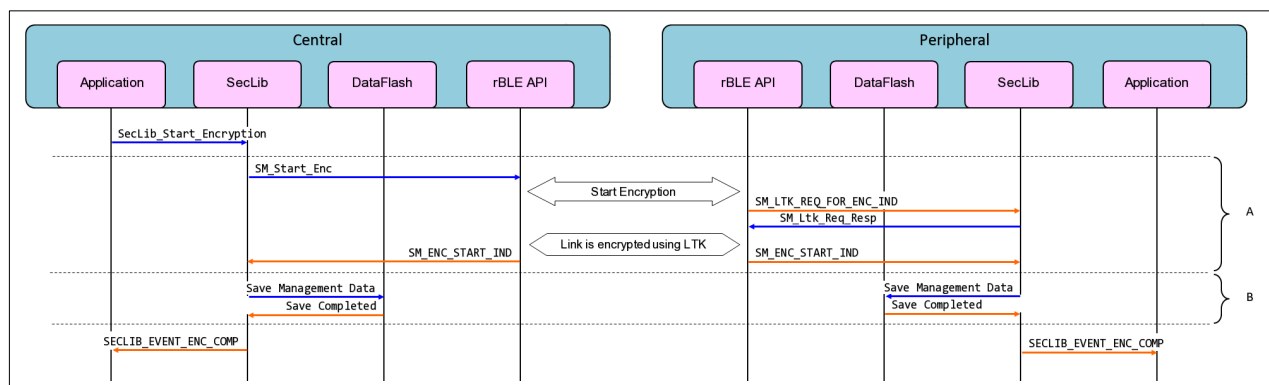
図 5-5 Central 開始暗号化シーケンス
