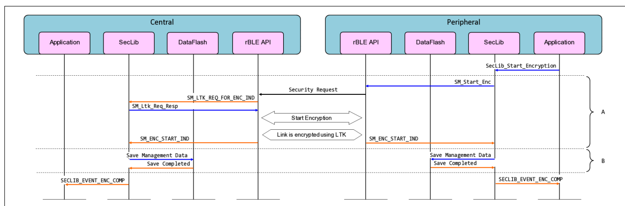
図 5-6 Peripheral 開始暗号化シーケンス
