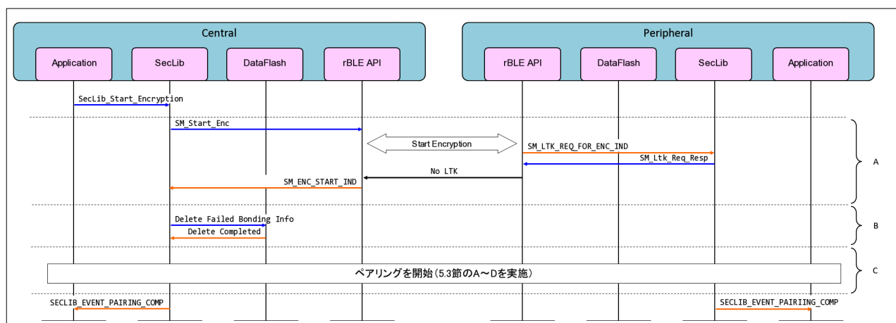
図 6-1 脆弱性のあるシーケンス
