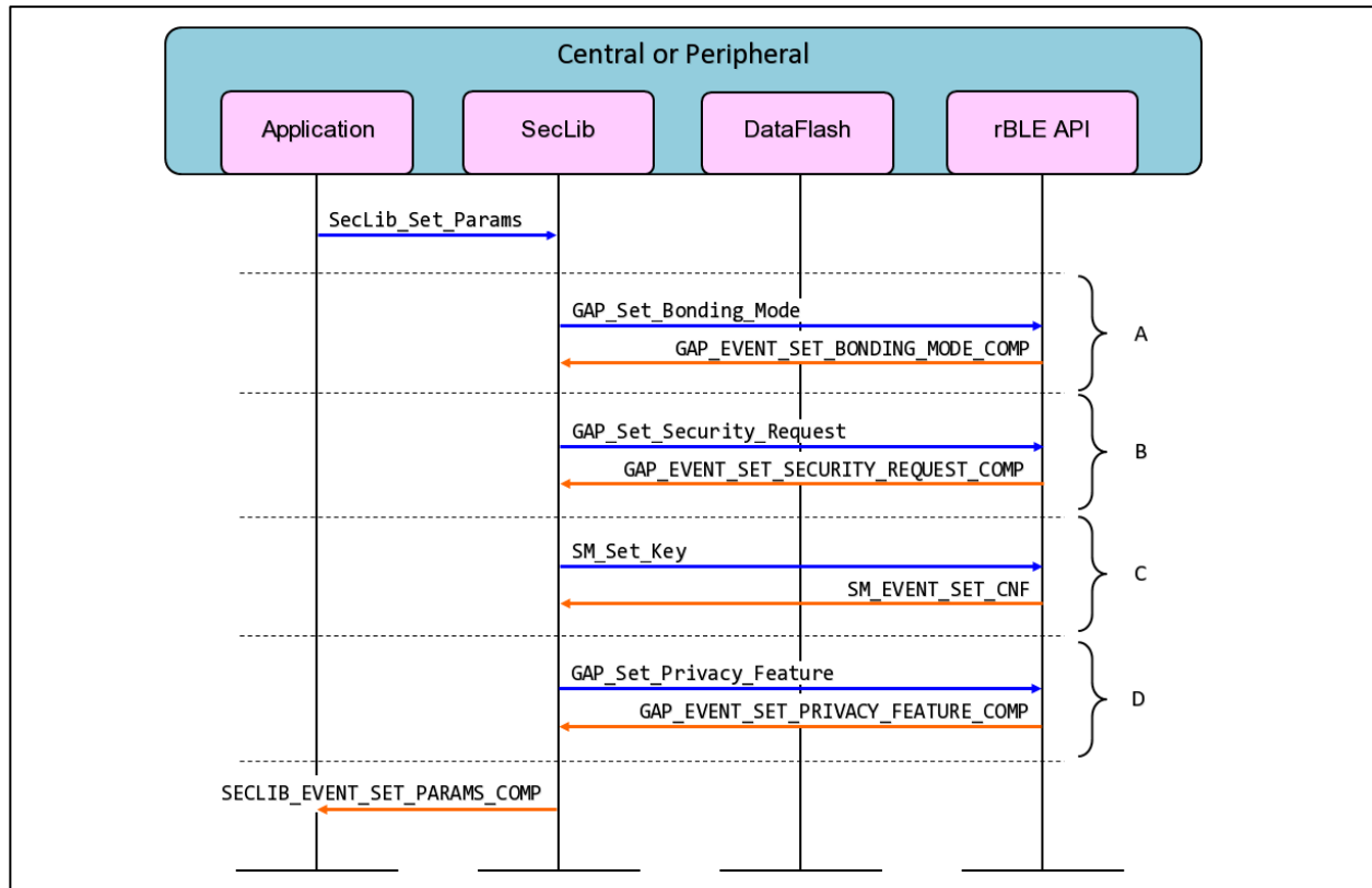
図 5-2 セキュリティパラメータ設定シーケンス
