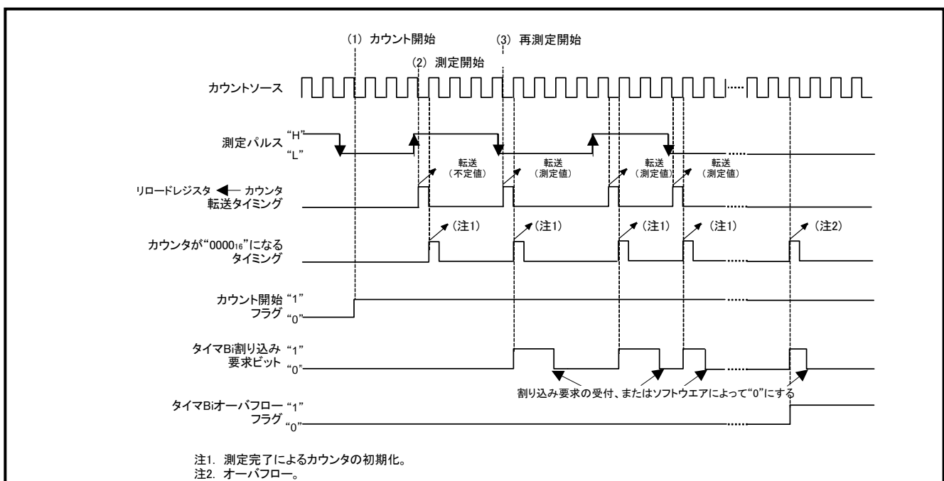
図 1. パルス幅測定モード動作タイミング図
